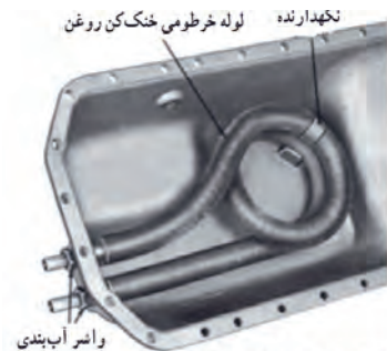
الف- عبور لوله مایع خنک‌کننده از کارتر ب- عبور مایع خنک‌کننده از پایه فیلتر JD314 ج- رادیاتور روغن U650 شکل ۴۶. انواع خنک‌کن روغن رایج در تراکتورها
