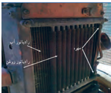
الف- عبور لوله مایع خنک‌کننده از کارتر ب- عبور مایع خنک‌کننده از پایه فیلتر JD314 ج- رادیاتور روغن U650 شکل ۴۶. انواع خنک‌کن روغن رایج در تراکتورها
