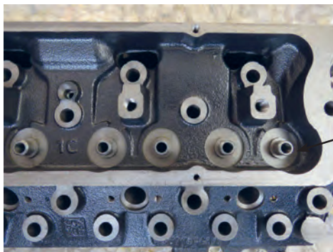
شکل ۱۶. گیت سوپاپ
