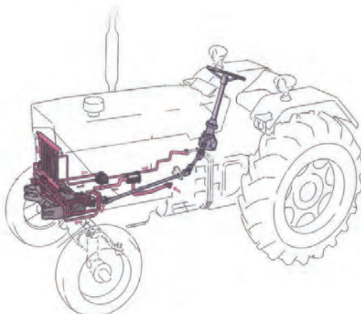
شکل ۱۷. مدار کامل فرمان نیمه هیدرولیک تراکتور U650
