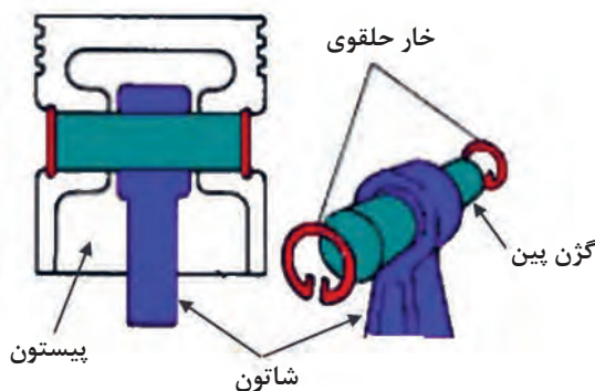
شکل ۱۵. اتصال شاتون به پیستون با گژن پین
