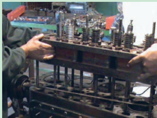
شکل ۴۸. برداشتن سرسیلندر
