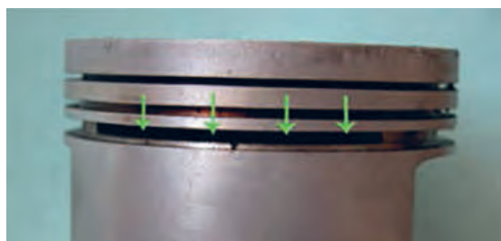
شکل ۹. ترتیب قرار گرفتن رینگها و موقعیت شیار عرضی پیستون زیر ناحیه قرار گرفتن رینگ روغنی
