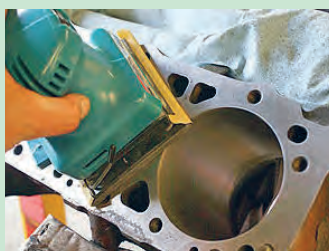
شکل ۶۶. تمیز کردن سطح بلوکه سیلندر با سنباده زن دستی و الکتریکی
