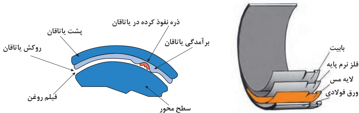
شکل ۱۹. انواع لایه بندی یاتاقان
