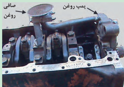
الف- محل پیچ‌های اتصال پمپ روغن به بلوک سیلندر
