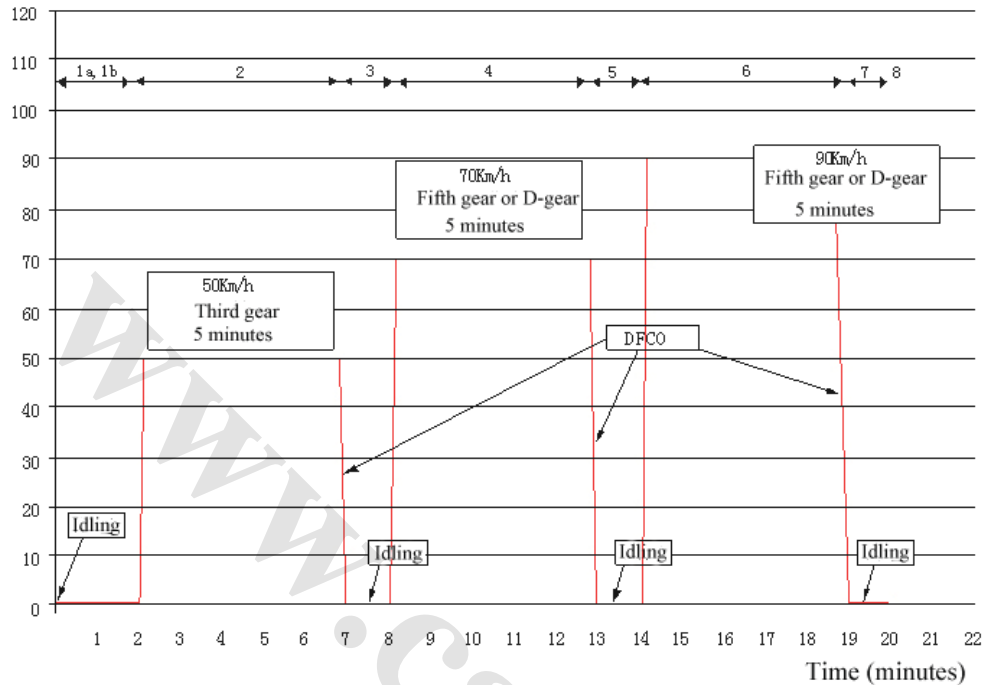
شکل ۱۷-۲ مراحل تست بعد از کشف کد نقص
