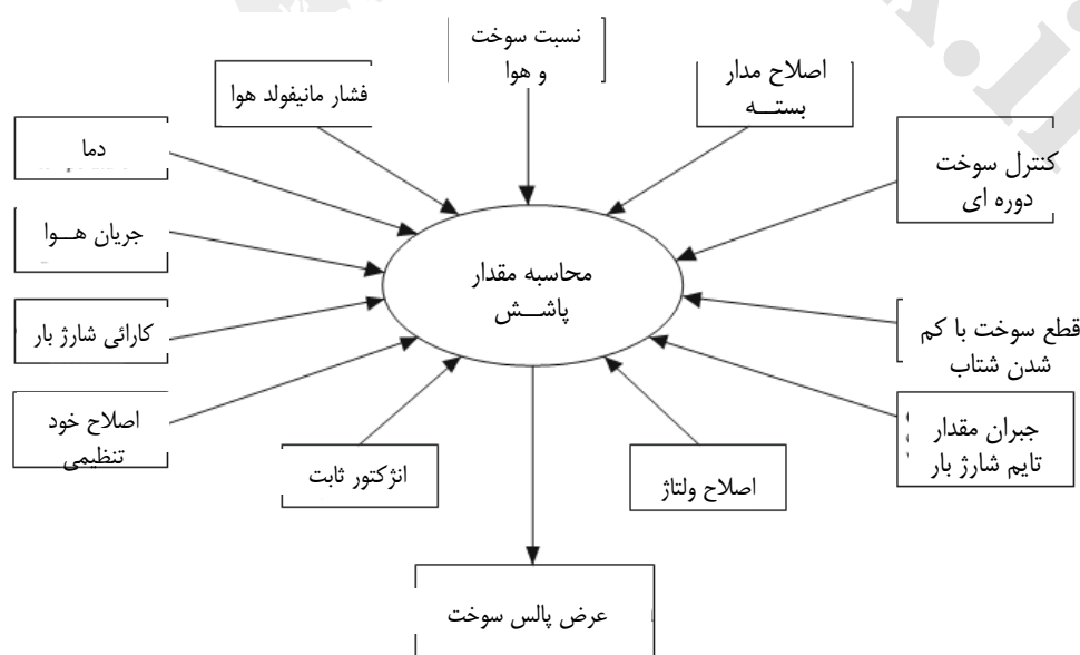
محاسبه عرض پالس پاشش سوخت : شکل ۱-۲
