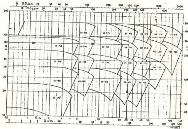
پمپ‌های CPK (جدول کلی انتخاب) دور n=2900 \text{ 1/min}
