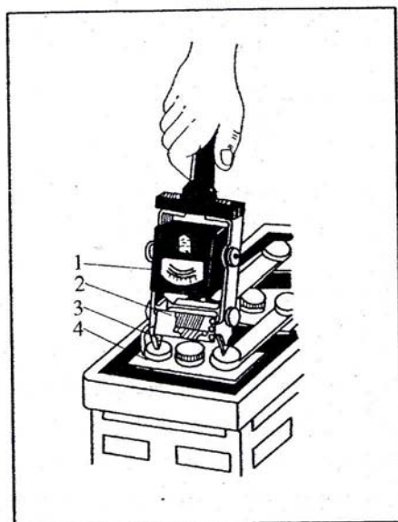
شکل ۱۰-۳: بررسی باتری با استفاده از چنگال شارژ-تخلیه باتری ۱. ولت‌متر، ۲. مقاومت، ۳. حسگر چنگال تخلیه، ۴. باتری
