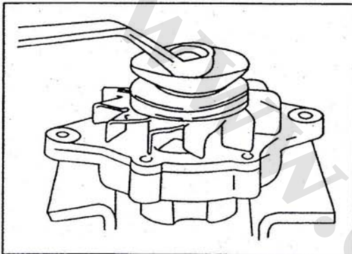
شکل ۱۰-۳-۴۳: نصب روتور
