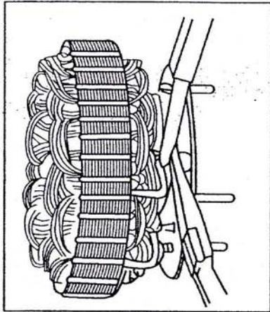
شکل ۱۰-۳-۴۲: نصب استاتور
