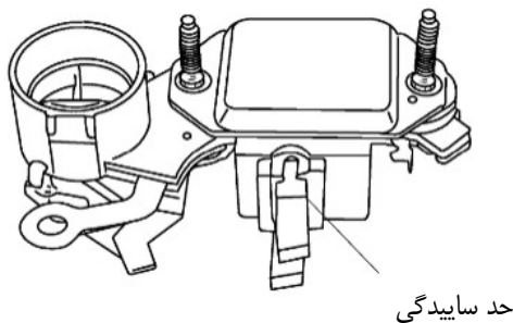
شکل ۳-۳۲: کنترل ذغال کربنی
