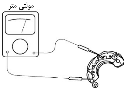
شکل ۳-۳۰: کنترل مدار بسته بین ترمینال ها
