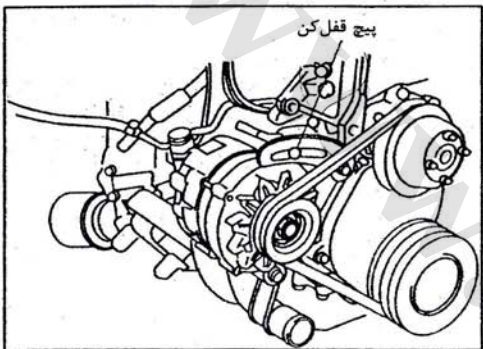
شکل ۱۰-۳-۱۰: نصب آلترناتور
