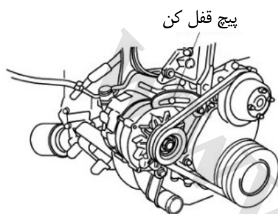
شکل ۳-۱۰: نصب آلترناتور
