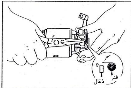
شکل ۱۱-۲-۱۰: در آوردن ذغال و پایه ذغال
