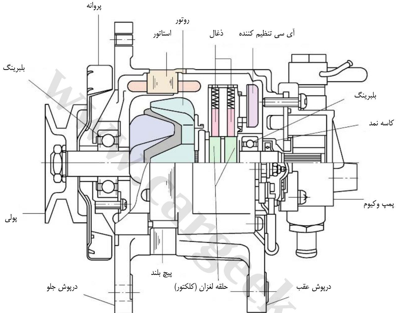
شکل ۱-۳: ساختمان دینام
