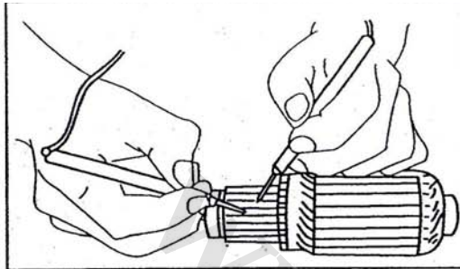
شکل ۱۰-۲۱: تست زمین آرمیچر
