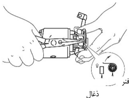
شکل ۲-۱۱: در آوردن ذغال و پایه ذغال
