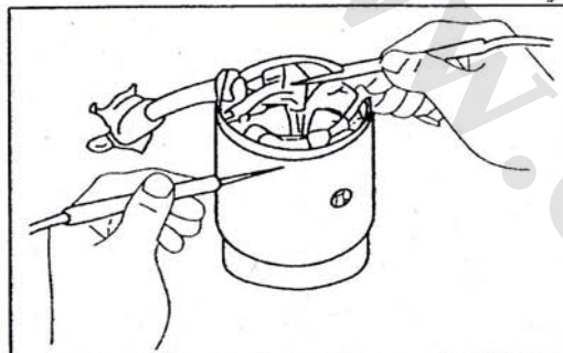
شکل ۱۰-۲۳: تست زمین سیم پیچ میدان مغناطیسی
