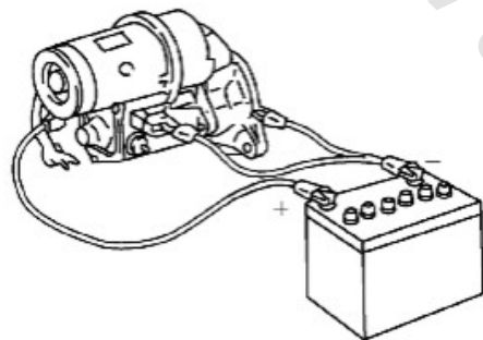
شکل ۲-۳۲: تست برگشت
