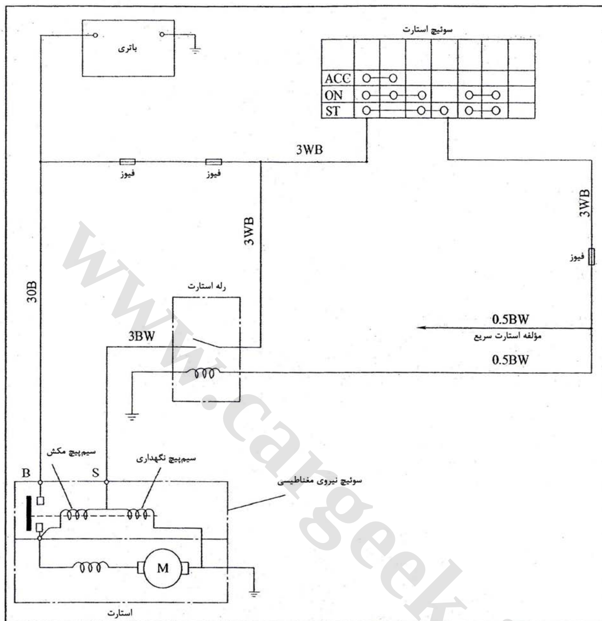
شکل ۱۰-۲-۳: سیم پیچ استارت
