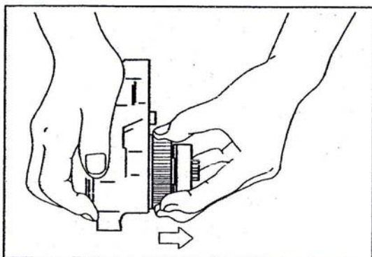
شکل ۱۲-۲-۱۰: درآوردن کلاچ جفجه‌ای
