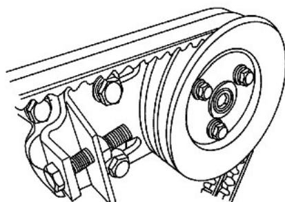
شکل ۳-۱۱: نصب مجموعه پمپ فرمان
