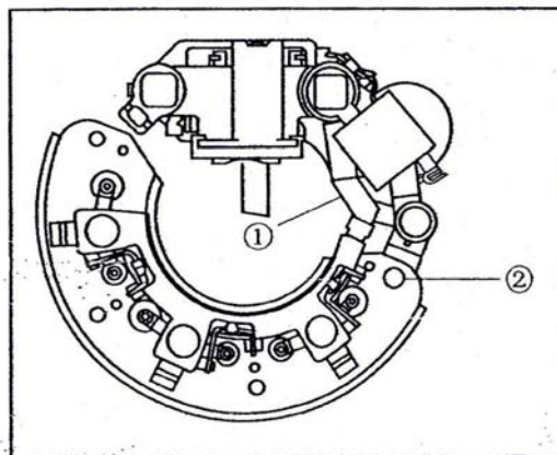
شکل ۴۱-۳-۱۰: نصب دیود
