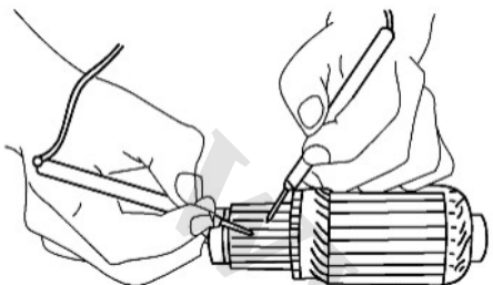
شکل ۲-۲۲: تست مدار بسته آرمیچر
