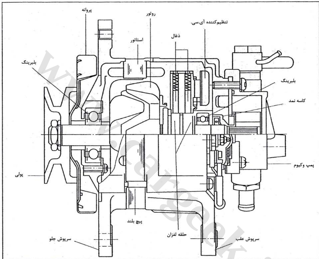
شکل ۱۰-۳-۱: ساختمان دینام
