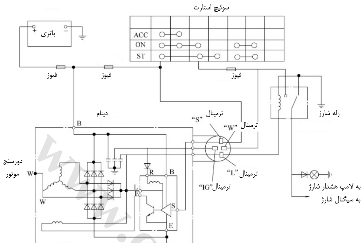
شکل ۳-۲: مدار شارژ
