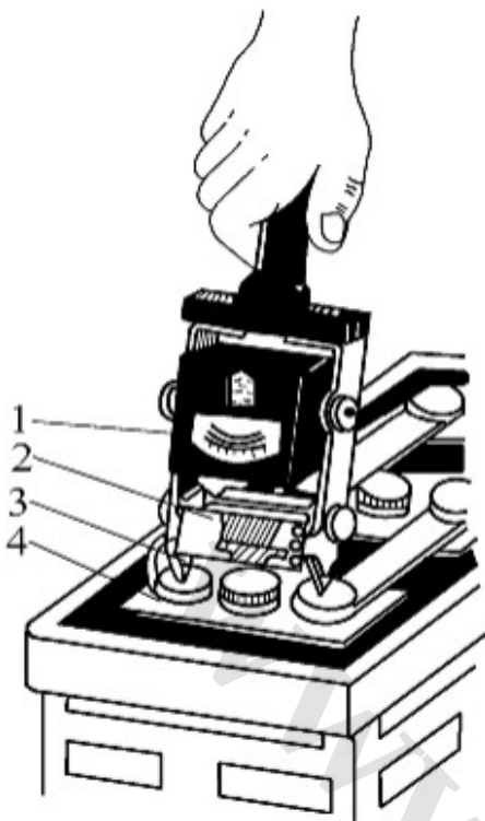
شکل ۱-۳: بررسی باتری با استفاده از چنگال شارژ-تخلیه باتری ۱. ولت‌متر، ۲. مقاومت، ۳. حسگر چنگال تخلیه، ۴. باتری
