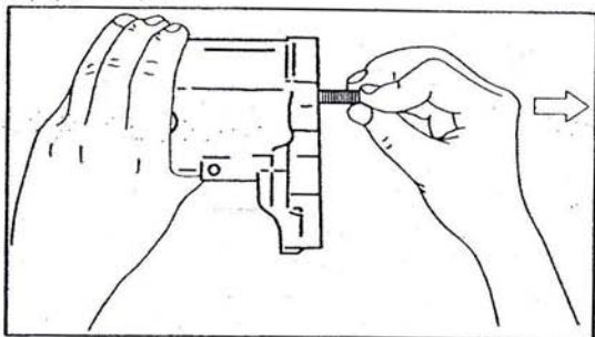
شکل ۱۰-۲-۱۳: پیاده‌سازی فنر برگشت سوئیچ مغناطیسی
