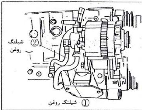
شکل ۱۰-۳-۱۳: نصب شیلنگ روغن
