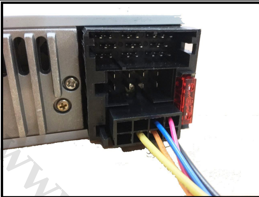
تصویر شماره ۶ - کانکتور تغذیه پشت رادیو CD در حالت مونتاژ شده
