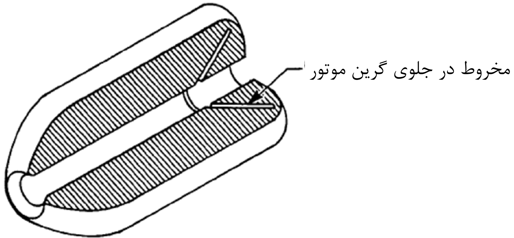
شکل ۵-۱۲ خرج استوانه‌ای مخروط‌دار
