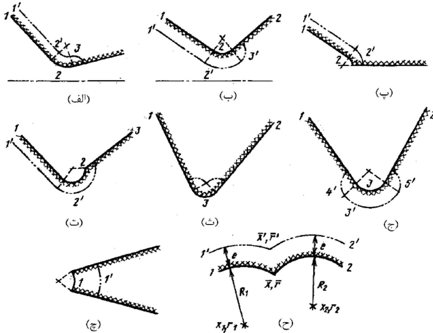
شکل ۵-۱۸ - شماهای سوزش قسمت‌های خرج پیشران:
