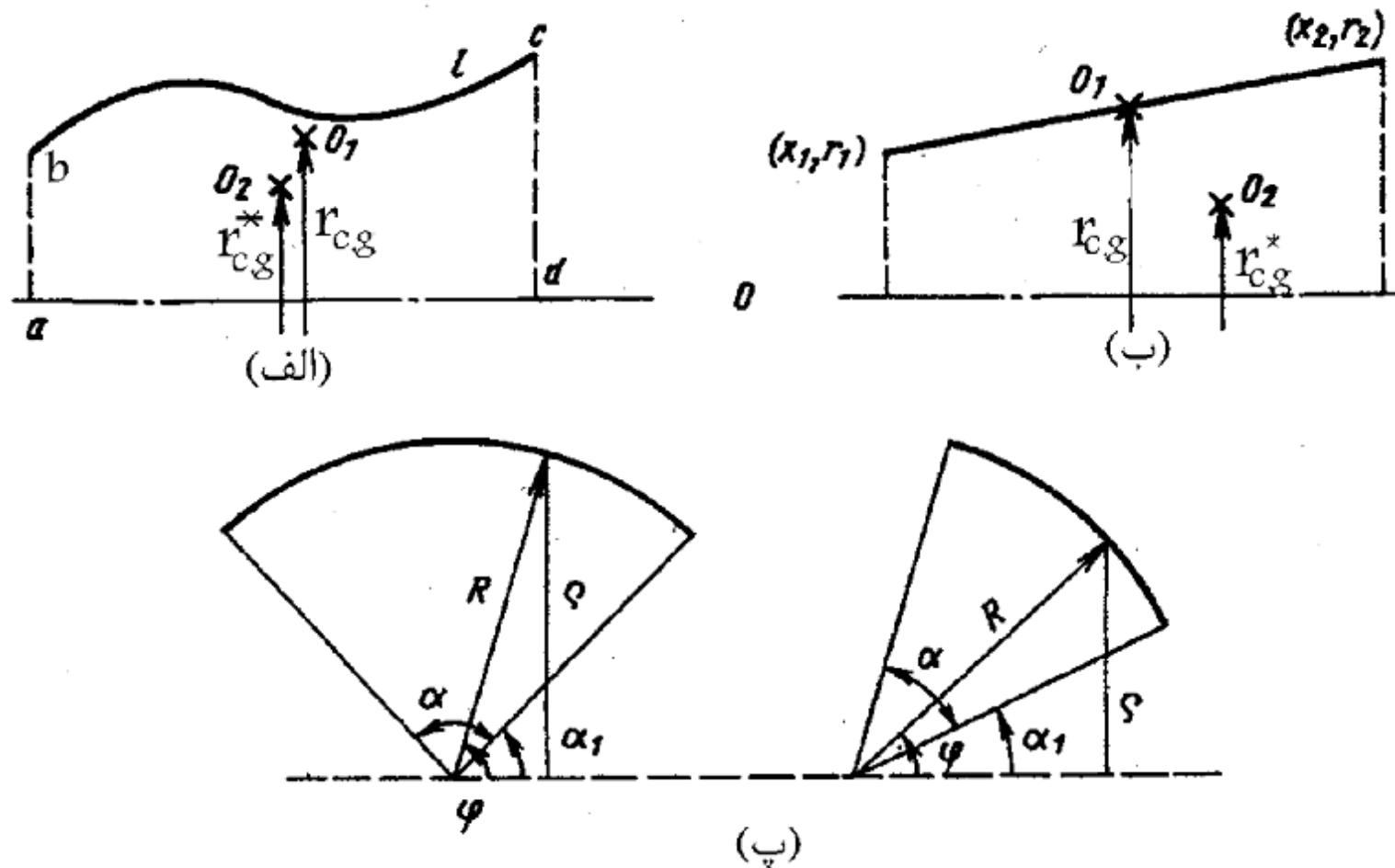
شکل ۵-۱۹- تئوری‌های مرتبط با اجسام حاصل از دوران
