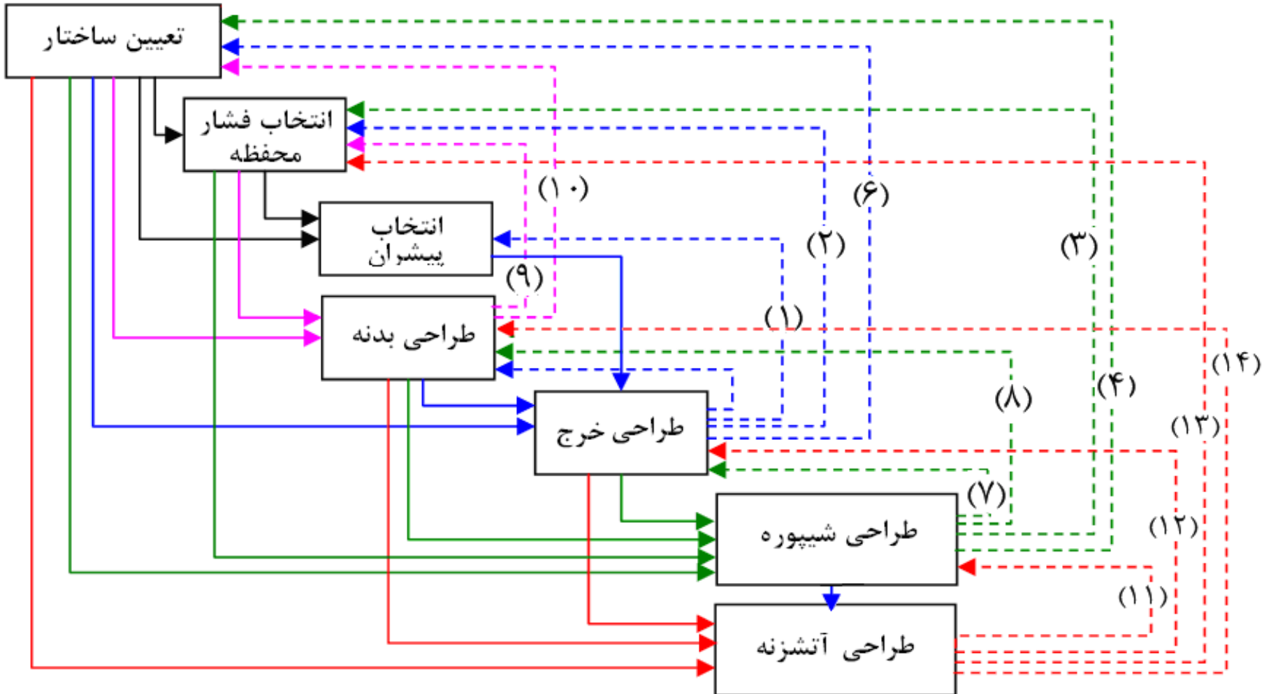
شکل ۴-۱ دیاگرام طراحی مفهومی موتور
