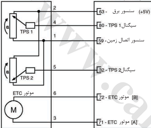
دیاگرام مدار ETC ماژول (CHG12)
