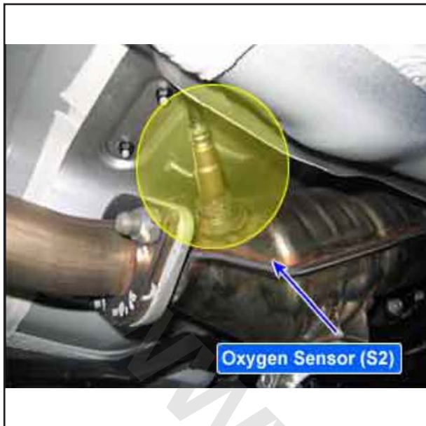
P۰۱۴۱ مدار گرمکن سنسور اکسیژن پایین دست (ردیف ۱/سنسور ۲) موقعیت سنسور اکسیژن پایین دست
