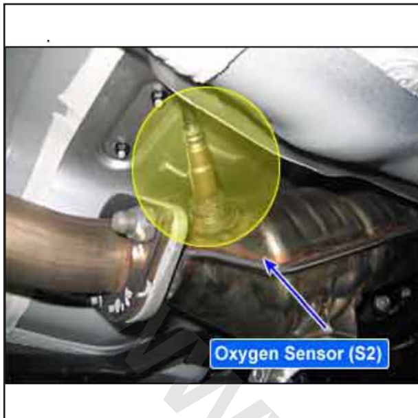
۳۸P۰۰ ولتاژ بالای مدار کنترل گرمکن سنسور اکسیژن پایین دست (ردیف ۱/سنسور ۲) موقعیت سنسور اکسیژن پایین دست
