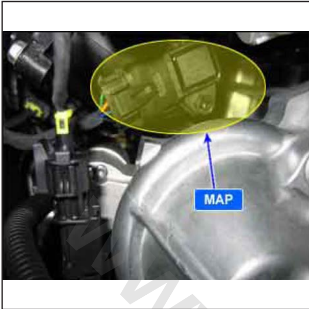
P۰۱۰۶ بازه / عملکرد فشار مطلق / فشار جوی منیفلد هوا موقعیت سنسور فشار منیفلد هوا
