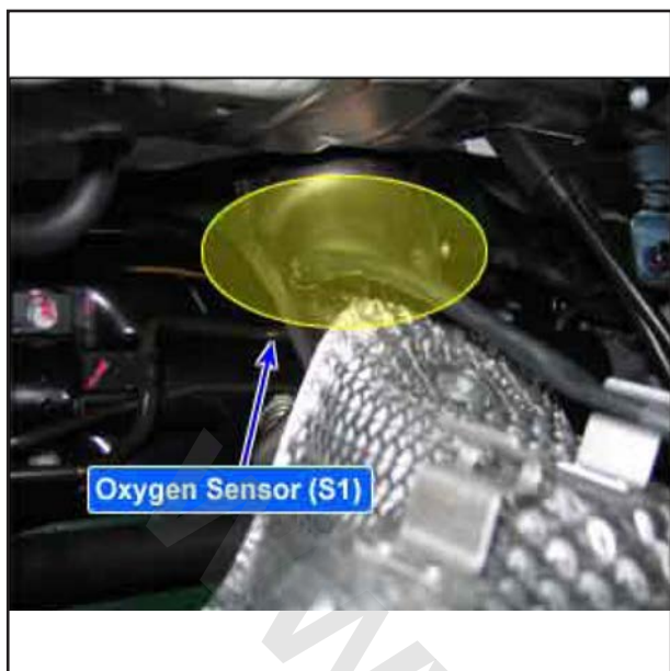
P۰۰۳۲ ولتاژ بالای مدار کنترل گرمکن سنسور اکسیژن بالادست (ردیف ۱/سنسور ۱) موقعیت سنسور اکسیژن بالادست
