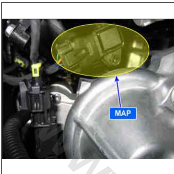
P۰۱۰۸ بالا بودن ولتاژ ورودی سنسور فشار مطلق / فشار جوی منیفلد هوا موقعیت سنسور فشار منیفلد هوا
