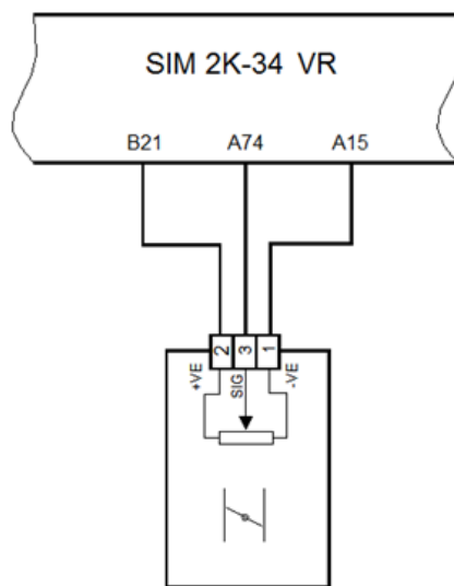
سنسور دریچه گاز
