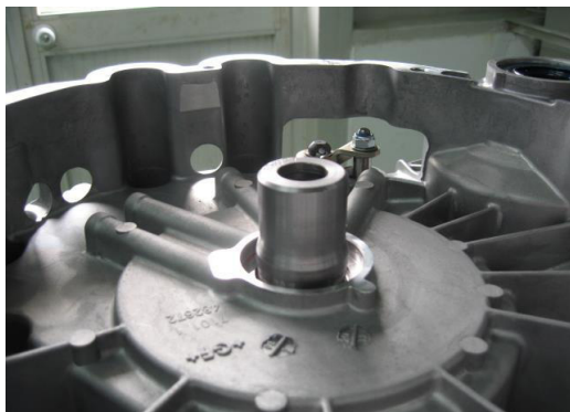
ابزار مخصوص را روی شفت ورودی قرار دهید (102971)
