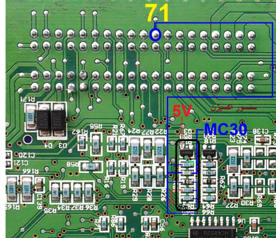
ورودی سیگنال سنسور اکسیژن
