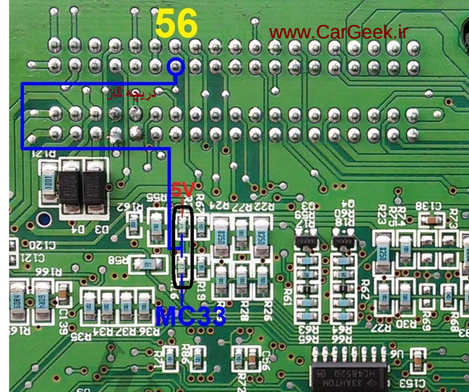
ورودی سیگنال سنسور درجه گاز
