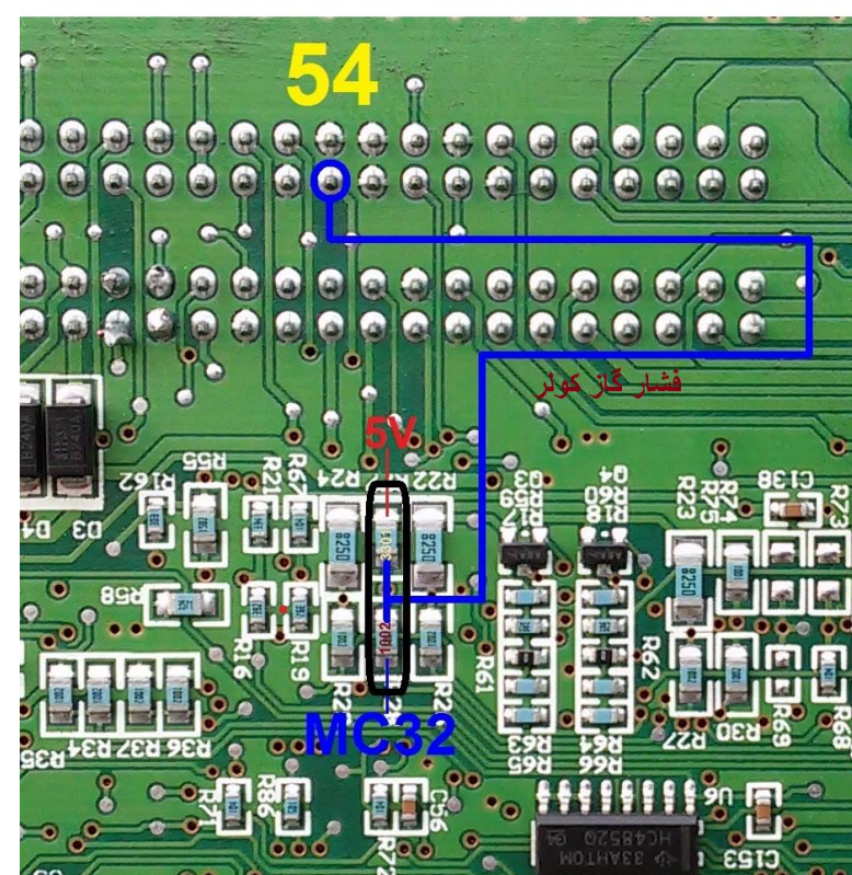
ورودی سیگنال سنسور فشار گاز
