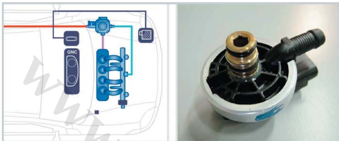
شکل ۱۵. انژکتورهای CNG
