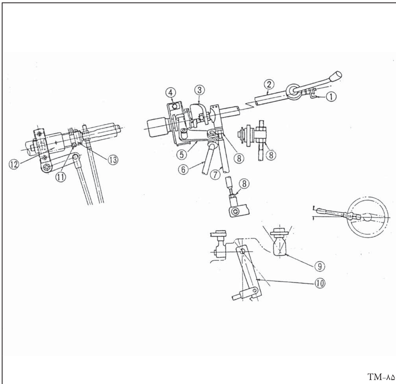
شکل TM-۸۵ مجموعه سیستم کنترل گیربکس
