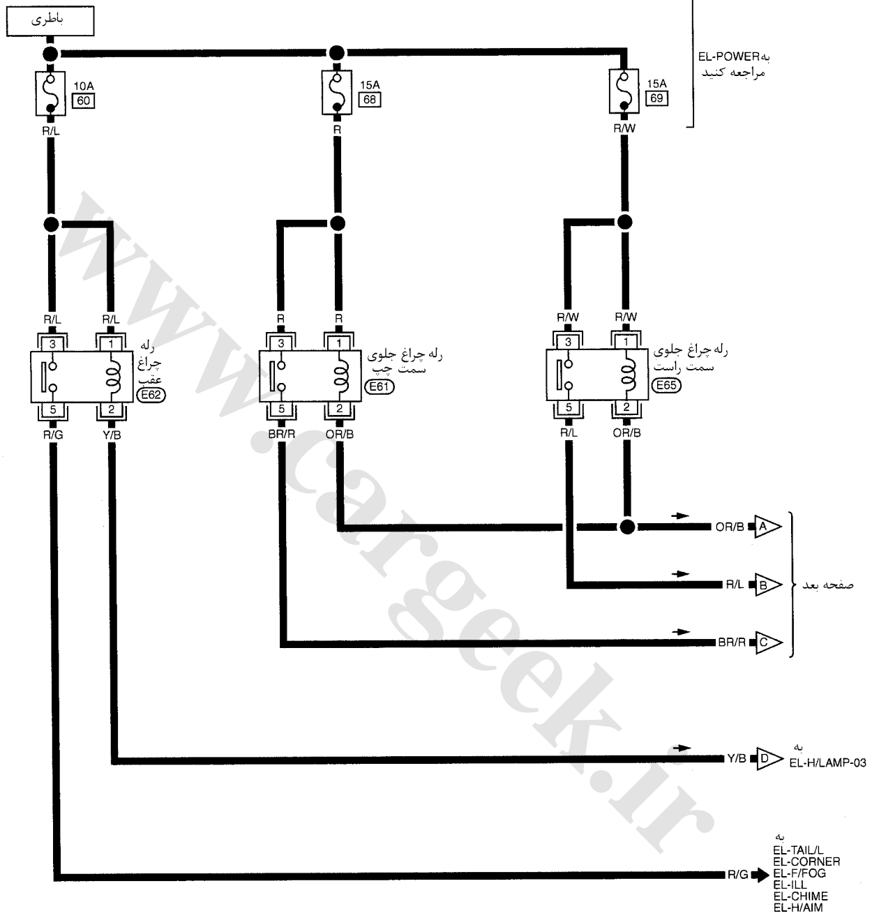
EL-H/LAMP-01
