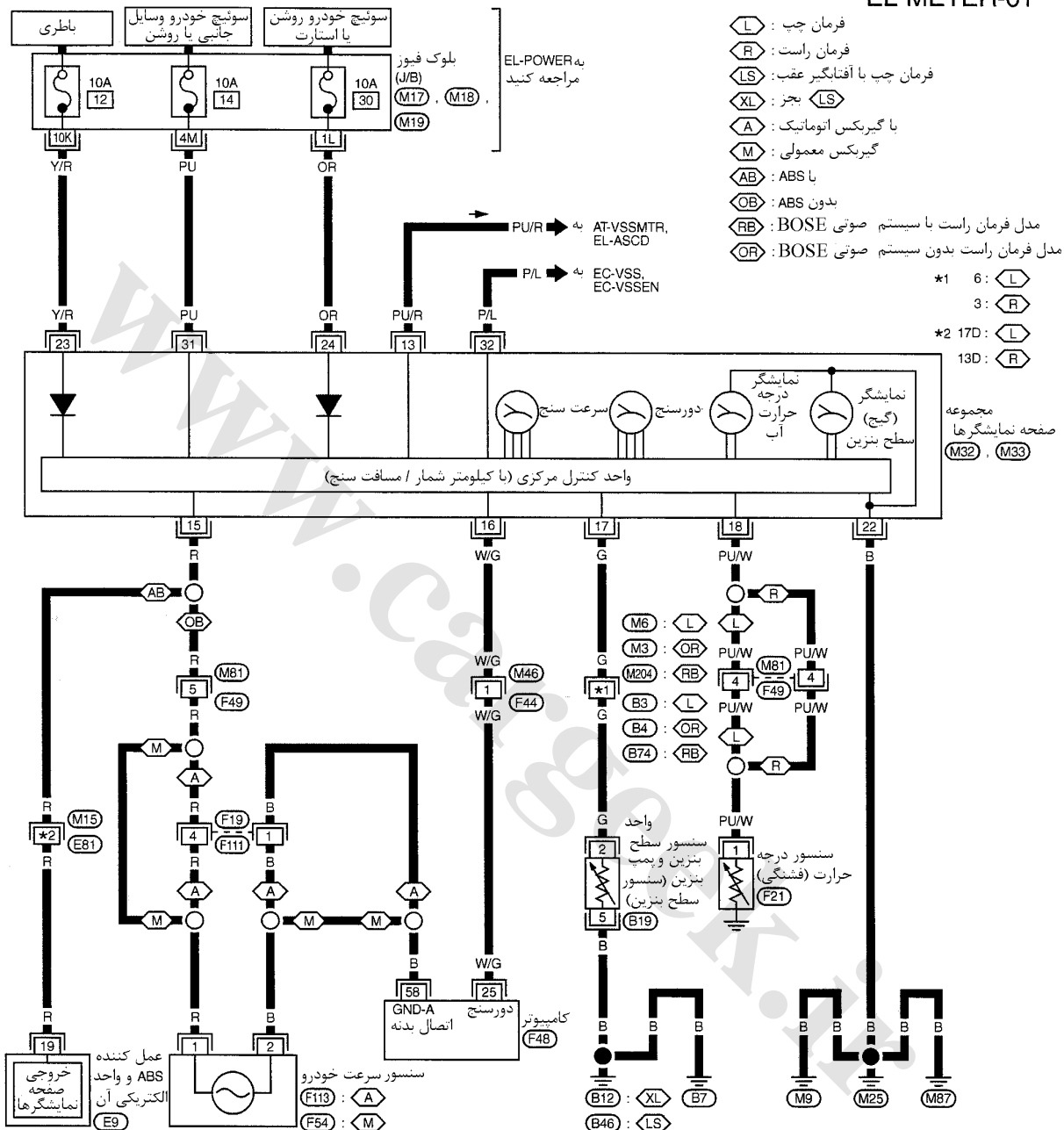
EL-METER-01
