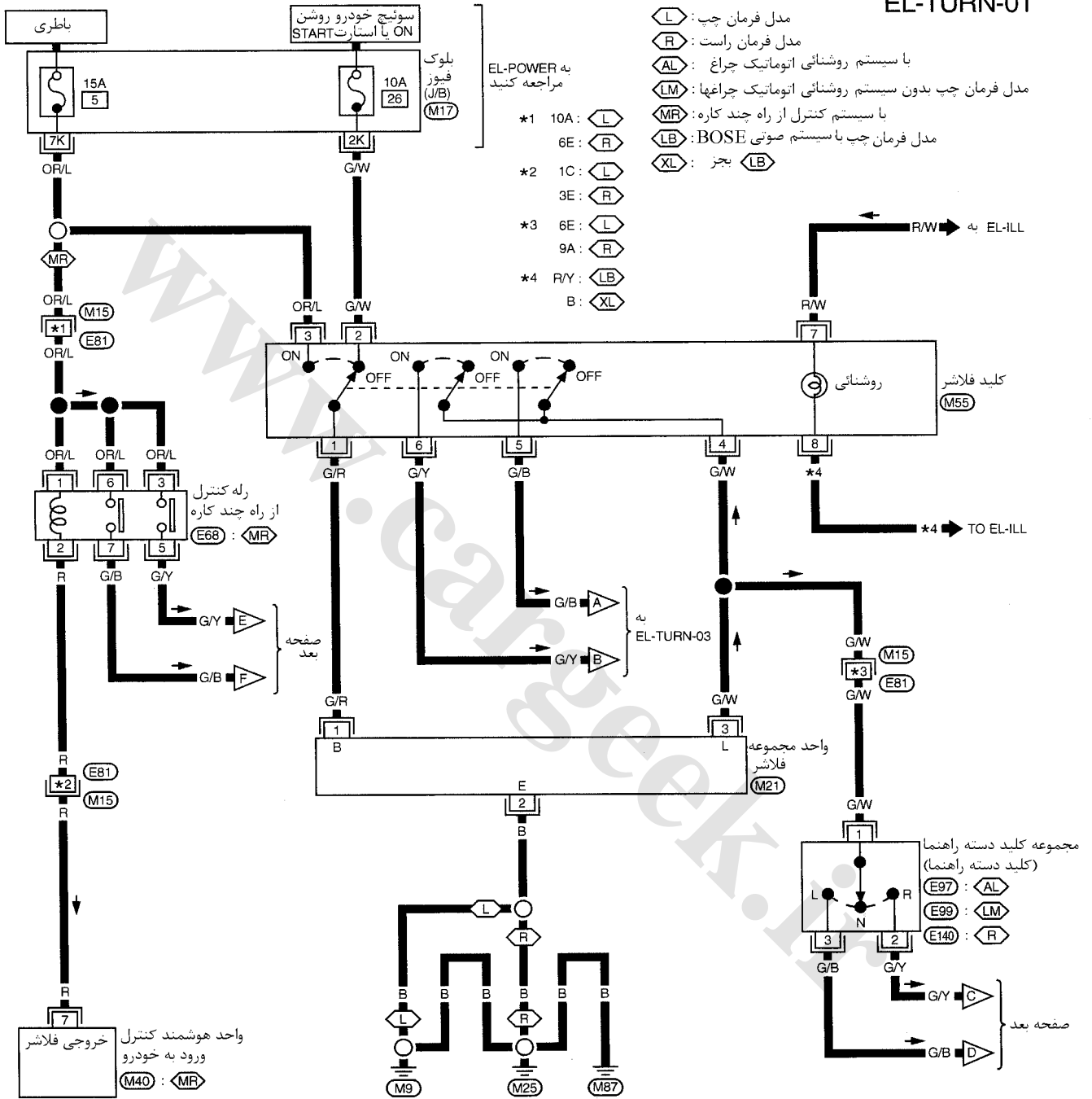
EL-TURN-01
