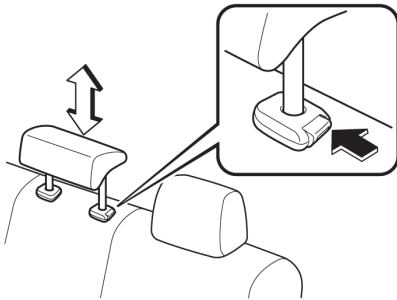
پیاده/سوار نمودن
