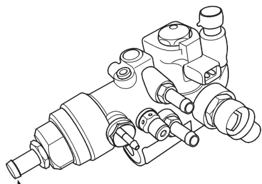
شکل ۵: رگلاتور فشار گاز
