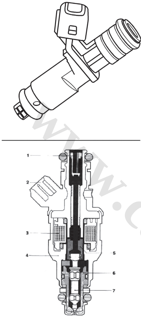
شکل ۱۲: انژکتور بنزین
