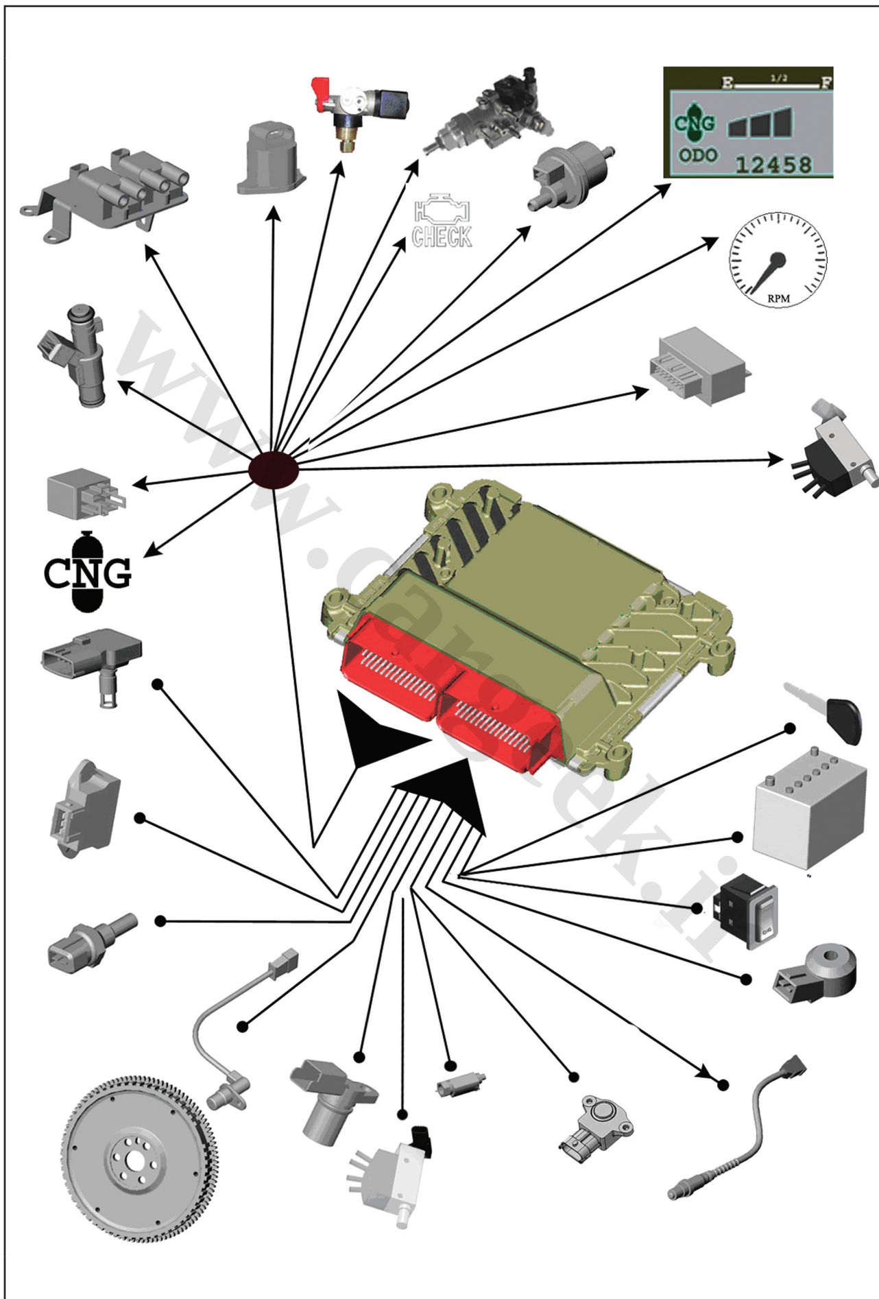
شکل ۲: سنسورها و عملگرهای مرتبط با ECU
