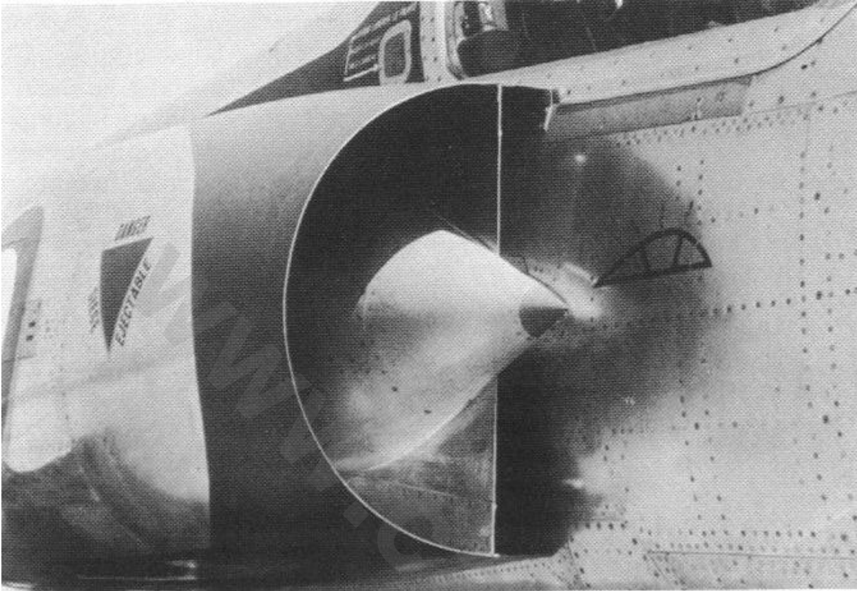
شکل ۳-۲۰ هواپیمای جنگی Mirage III با نصب کناری دیفیوزر های ضربه مایل
