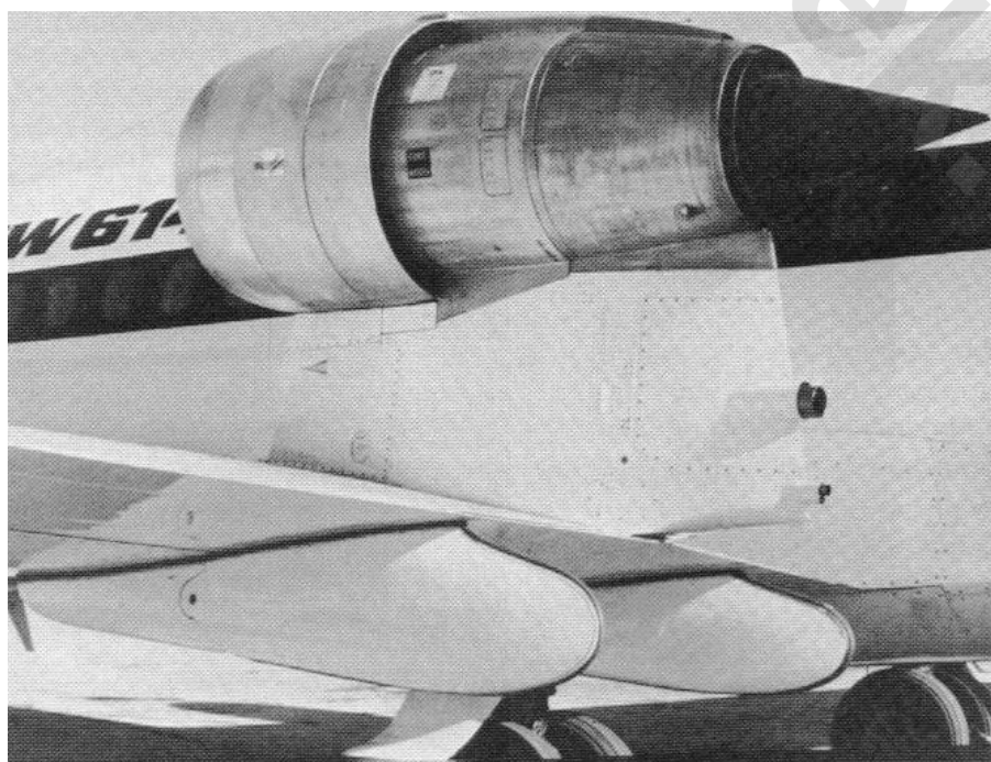
شکل ۶-۱۱ اولین هواپیما دارای نصب بالای بال (VFW-Fokker 614 در دهه ی شصت)
