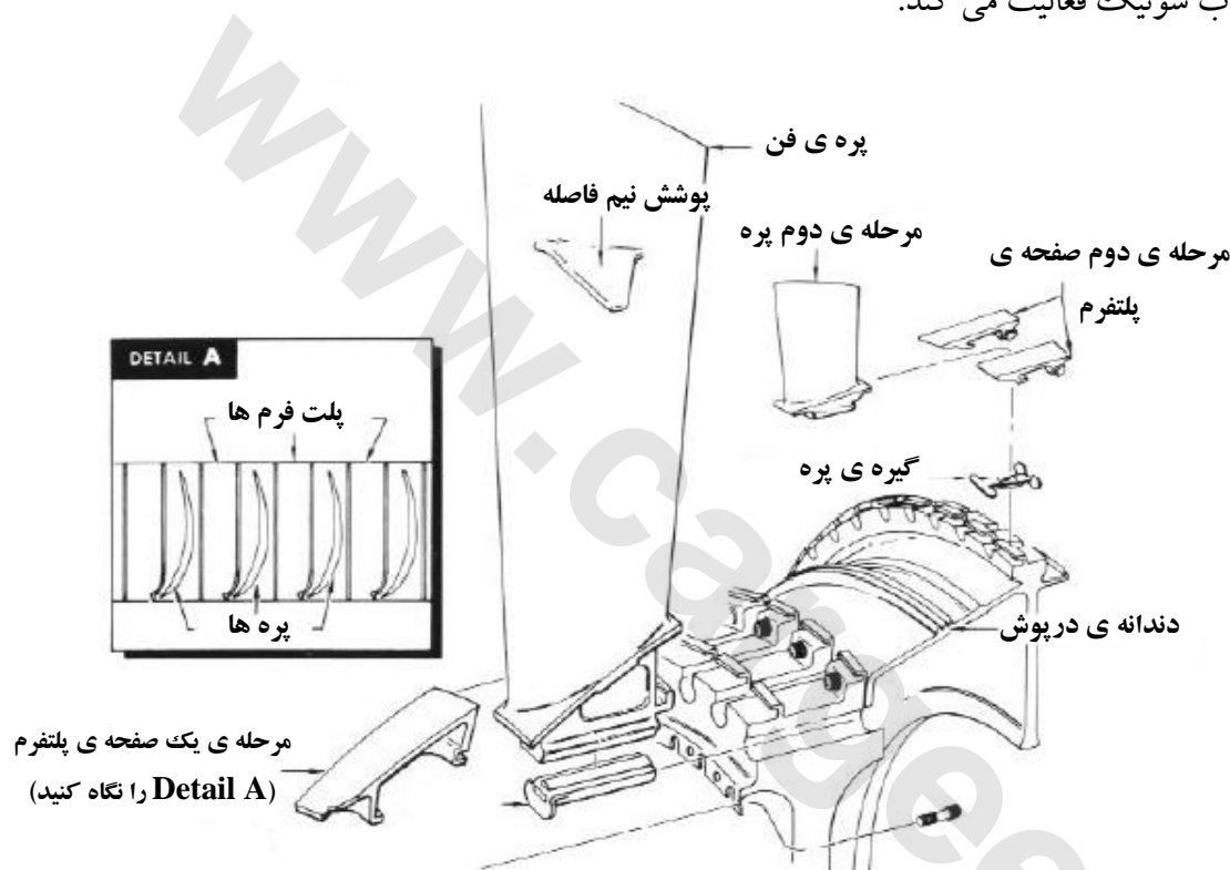
شکل ۴.۲۹ مونتاژ پره ی فن به صفحه ی روتور (موتور 6 CF6 ژنرال الکتریک)
