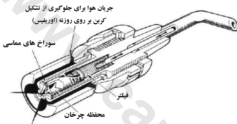
شکل ۹-۵ محفظه ی سوخت ساده (آتشیان)
