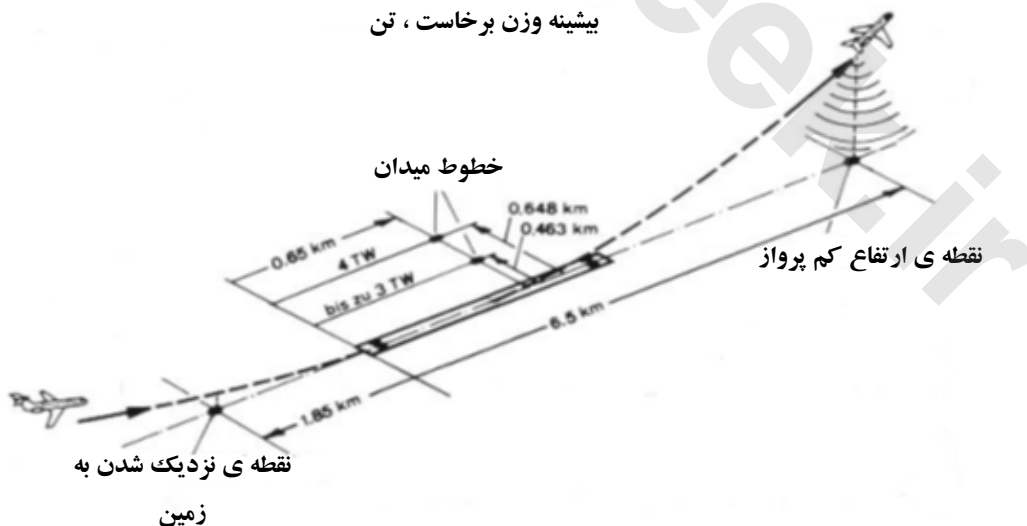
شکل ۱-۱ مقررات سرو صدا ی FAR 36
