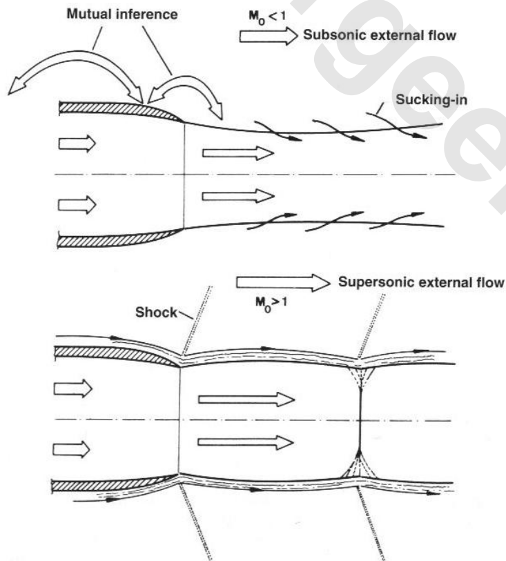
شکل ۱۱-۱۲ تأثیرات تداخلی بین خروجی جت و بدنه عقب هواپیما در سرعت پرواز سوپر سونیک و ساب سونیک
