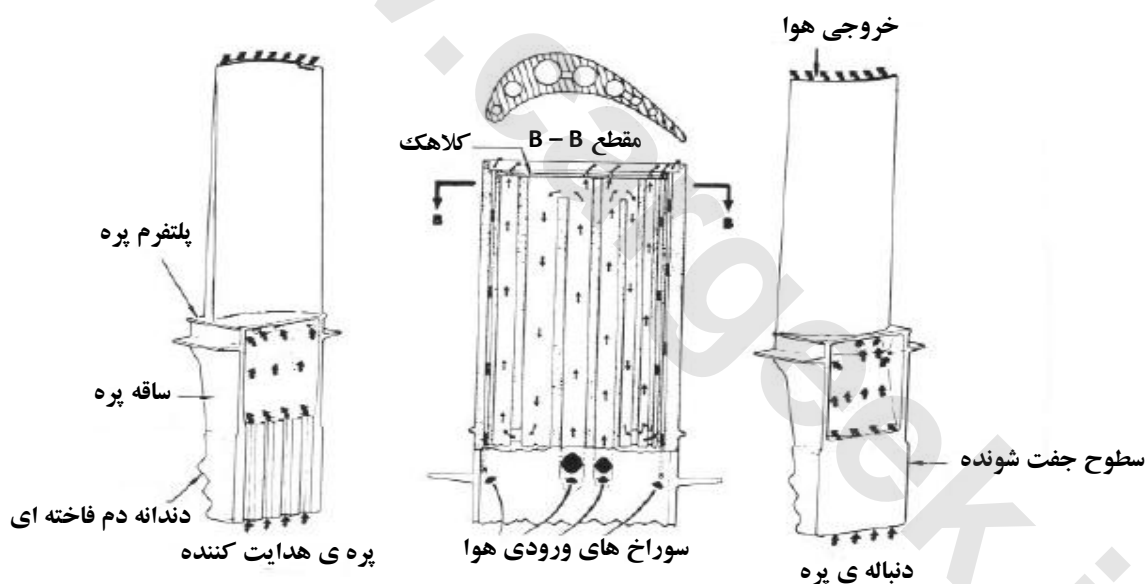
شکل ۹-۶ جزئیات خنک کنندگی پره ی توربین (مرحله ی دوم توربین فشار بالا ، CF6 ژنرال الکتریک)
