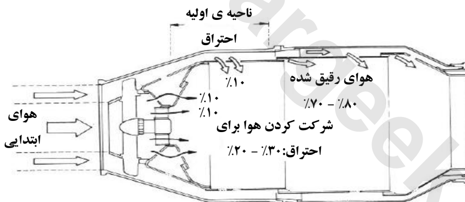
شکل ۲-۵ شمای جریان در اتاق احتراق
