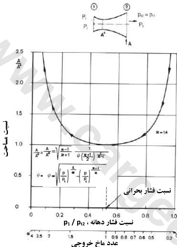
شکل ۷-۶ دهانه ی جریان گاز ایده آل
