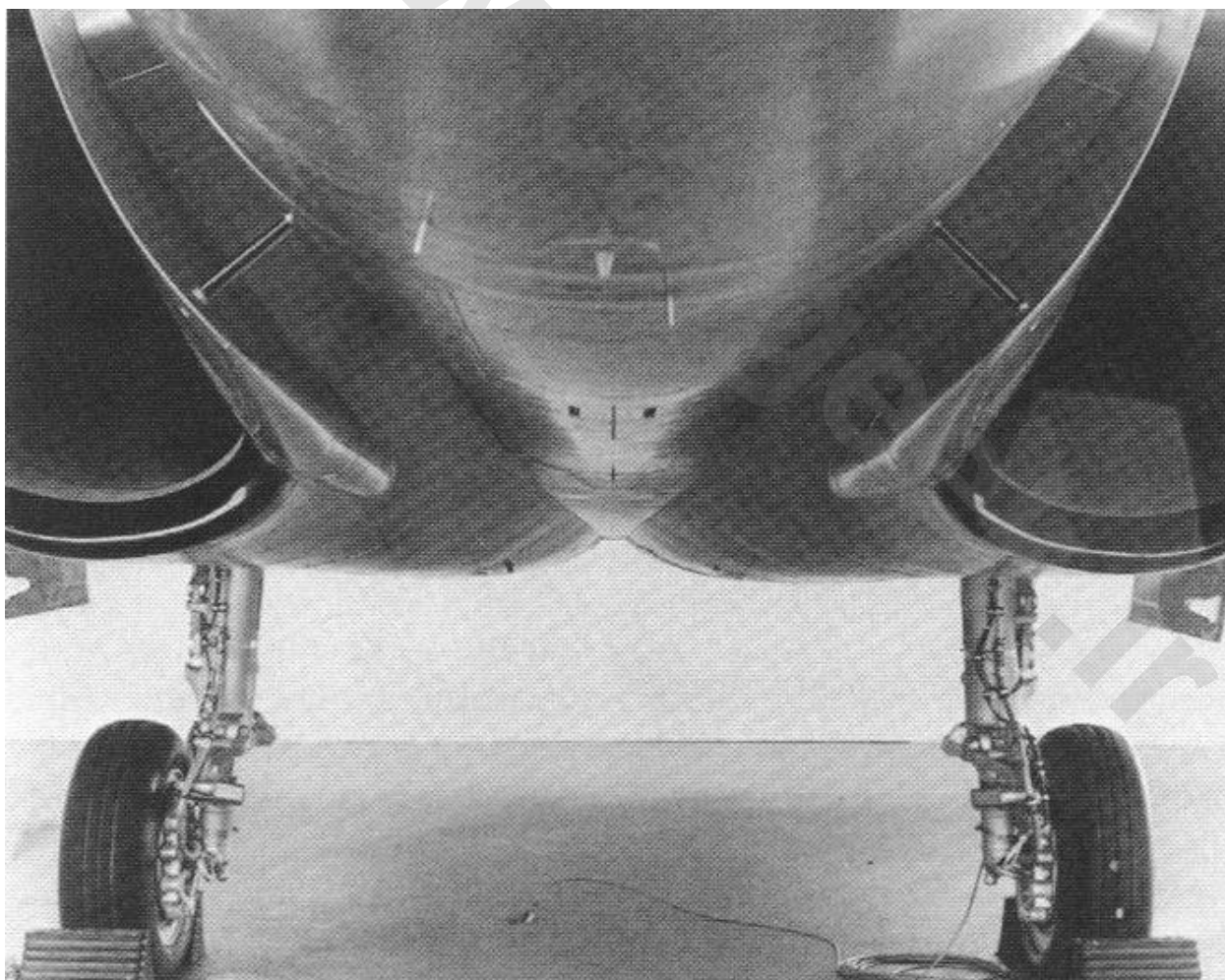
شکل ۱۸-۳ نمونه ی اصلی هواپیمای جنگی سبک وزن YF-17 با دیفیوزر های ضربه عمودی. صفحه های شکاف دار روی سمت دماغه ی هواپیما برای نگهداری لایه مرزی دماغه هواپیما از داخل شدن در ورودی ها
