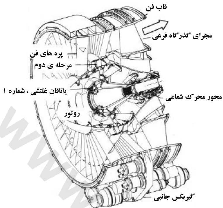
شکل ۴۲۷ بخش فن یک موتور کنار گذاری بالا (CF6 6 ژنرال الکتریک)
