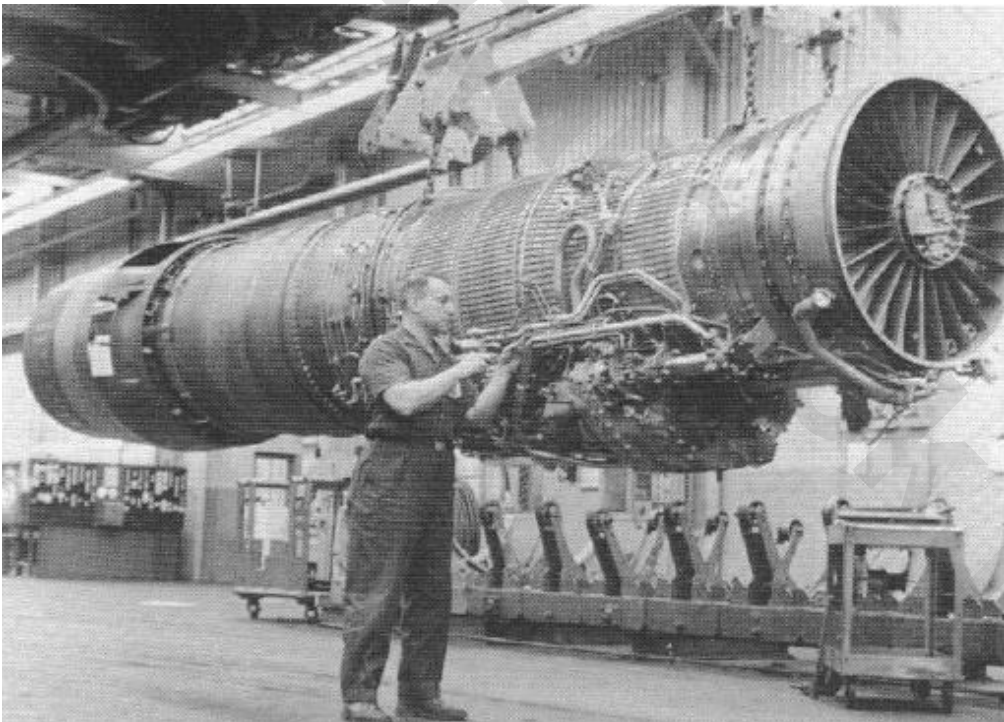
شکل ۱-۱۲ توربوفن Pratt & Whitney TF30-P-7 (نیروی ۹۲۰۰daN، کمپرسور ۱۶ مرحله ای، توربین ۴ مرحله ای، نسبت فشار کمپرسور ۱:۱۷.۵)
