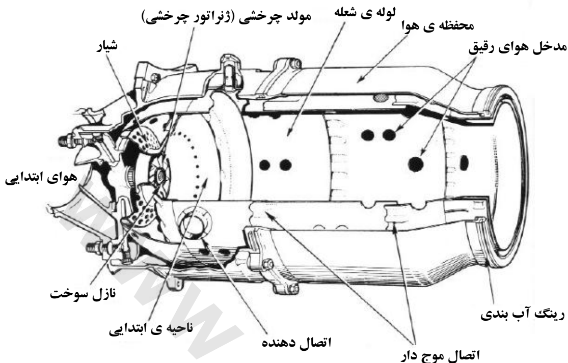
شکل ۱-۵ نمونه ای از مجموعه ی سوخت پاش
