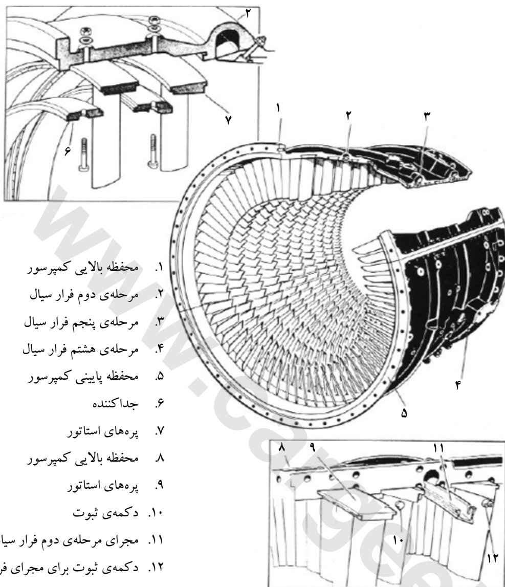
شکل ۴۶ محفظه کمپرسور (توربوجت اورند۱۴۱)
