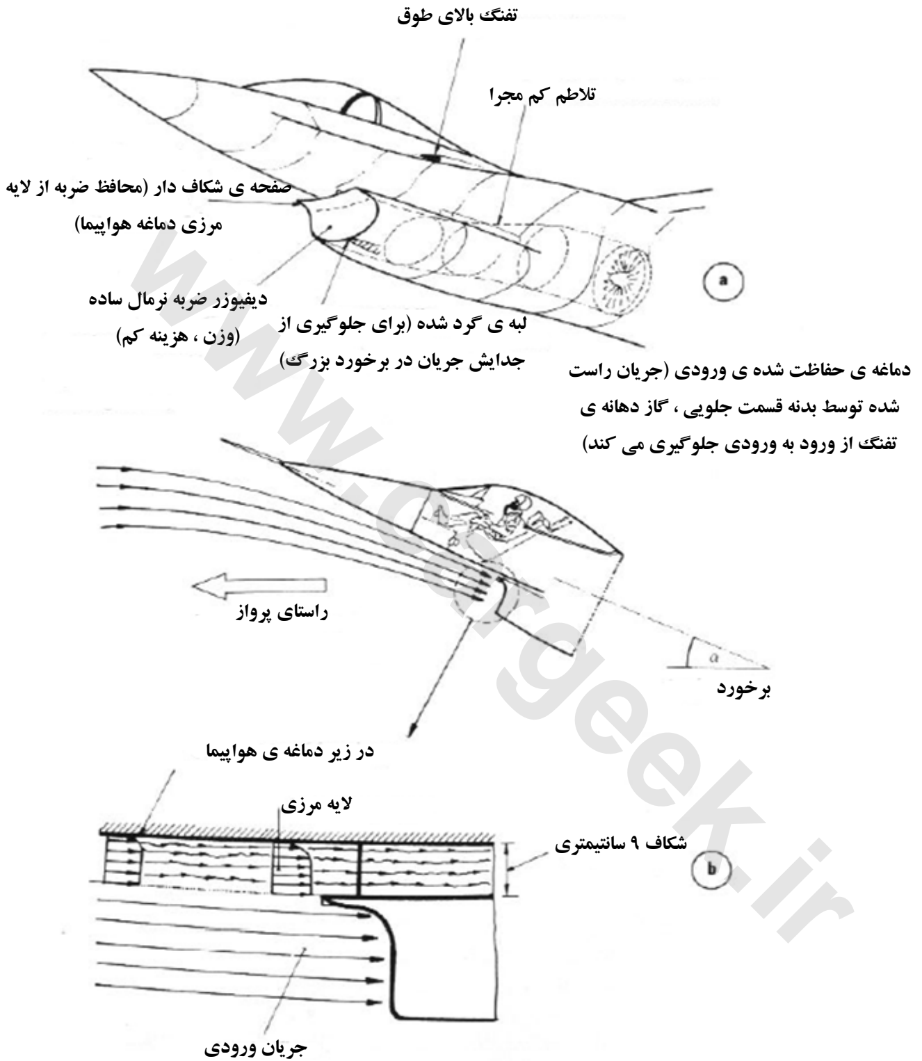
شکل ۱۷-۳ خصوصیات دیفیوزر ضربه عمودی F-16
