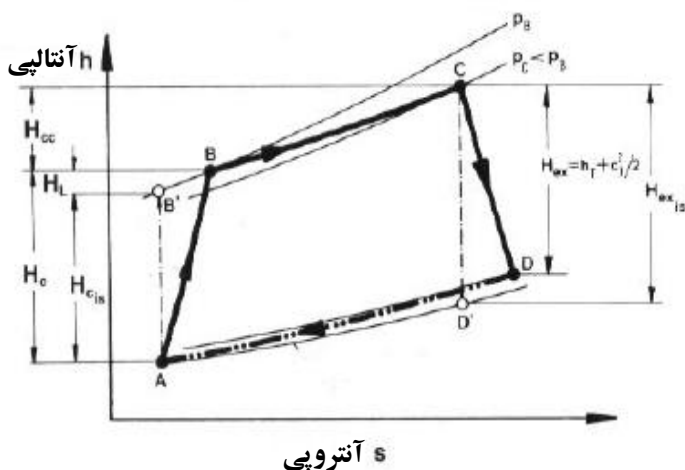
شکل ۲-۲ سیکل کاری توربین گازی در نمودار فشار - حجم و آنتالپی - آنتروپی.
