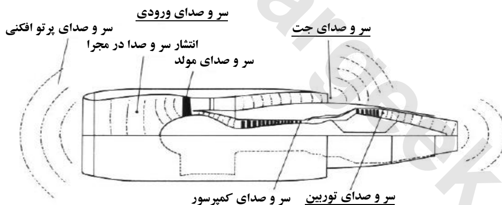
شکل ۱۰-۲ منابع سر و صدای درونی
