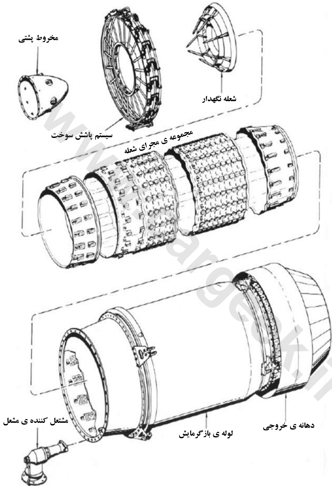
شکل ۴-۸ مجموعه ی پس سوز (General Electric J79)
