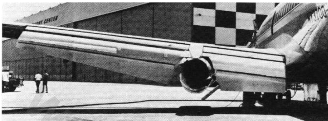
شکل ۳-۱۱ با نصب مستقیم موتور ها در زیر بال ، برش فلپ لازم می باشد
