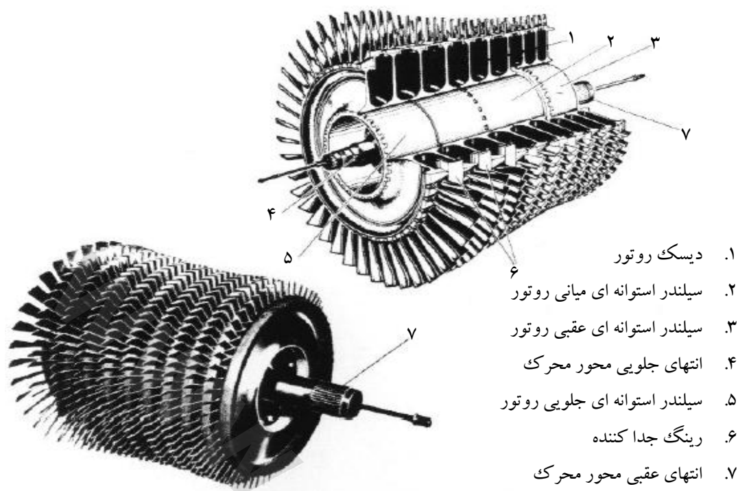
شکل ۴۹ روتور کمپرسور (موتور توربو جت Orenda 14)
