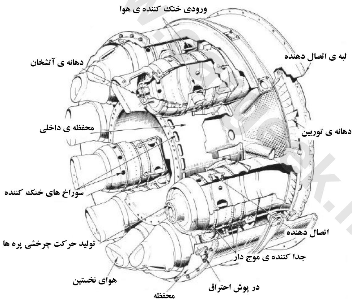
شکل ۵-۸ اتاق احتراق لوله مجزای حلقوی
