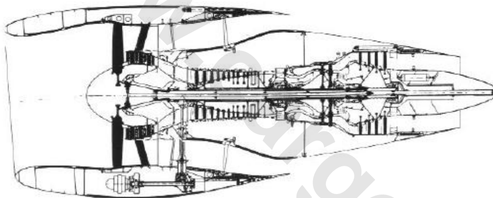
شکل ۲۰-۱ توربوفن General Electric CF6-50A با نسبت کنارگذاری بالا، با ترکیب سه تقویت کننده مرحله ی جریان پایین فن (پیشراشه ی ۲۲۲۰۰ daN، نسبت کنارگذاری ۵:۱، نسبت فشار کمپرسور ۱:۲۸.۴)
