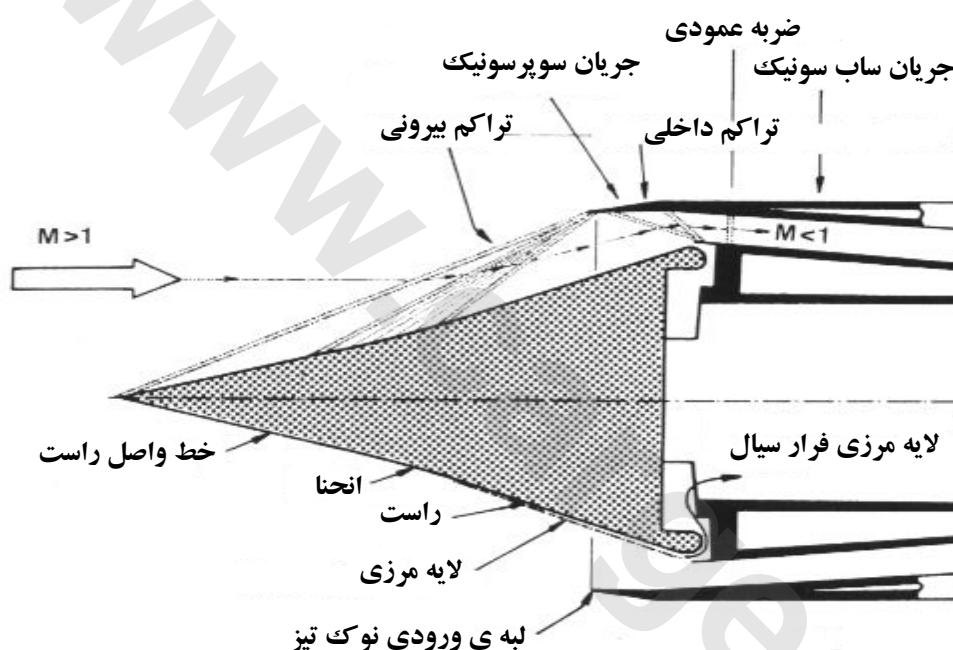
شکل ۲۲-۳ ورودی مرکب تراکم (Lockheed SR-71)
