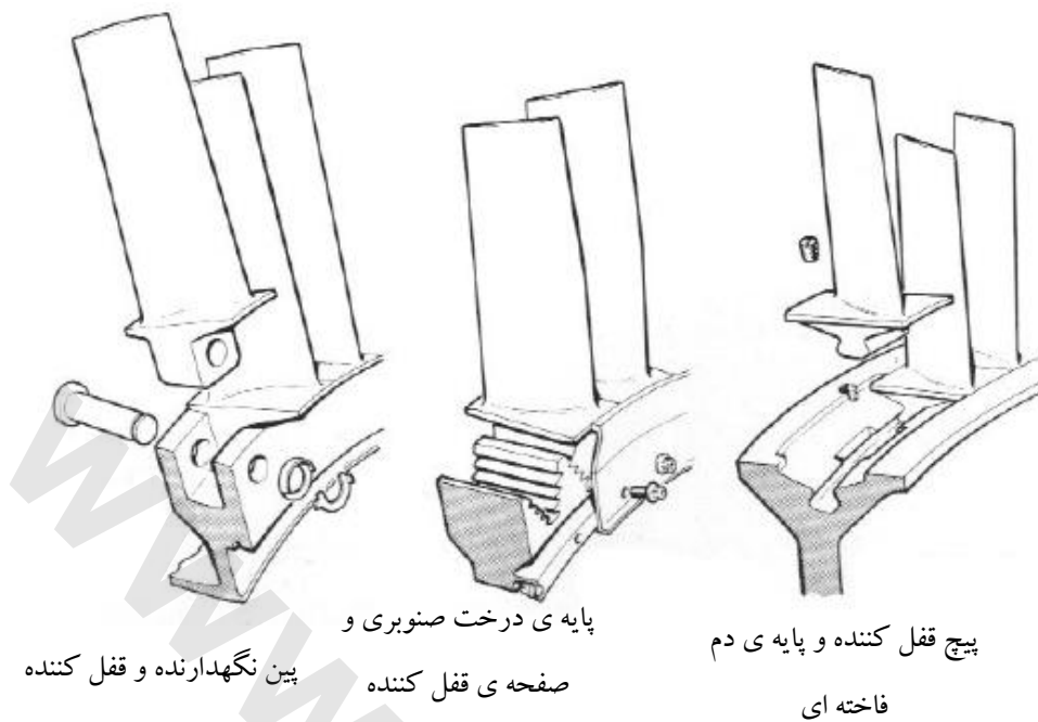
شکل ۴۱۱ روش های محکم کردن پره های روتور به دیسک
