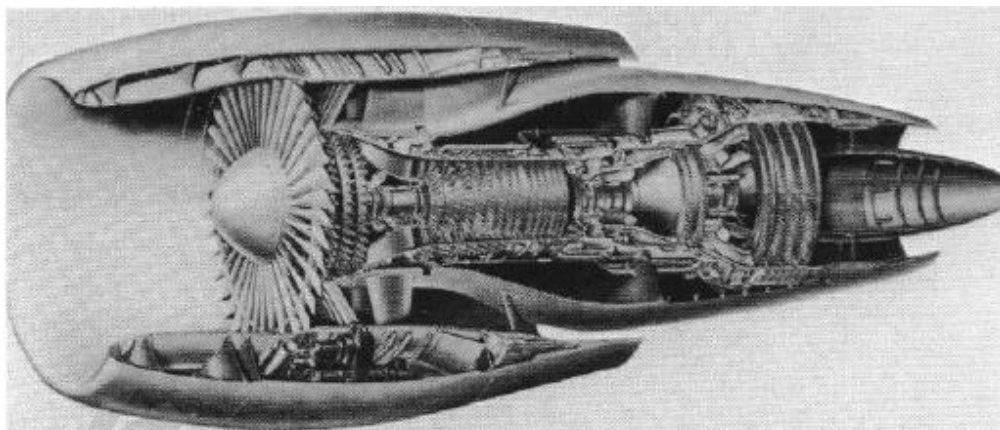
شکل ۲۰-۱ توربوفن General Electric CF6-50A با نسبت کنارگذاری بالا، با ترکیب سه تقویت کننده مرحله ی جریان پایین فن (پیشراشه ی ۲۲۲۰۰ daN، نسبت کنارگذاری ۵:۱، نسبت فشار کمپرسور ۱:۲۸.۴)
