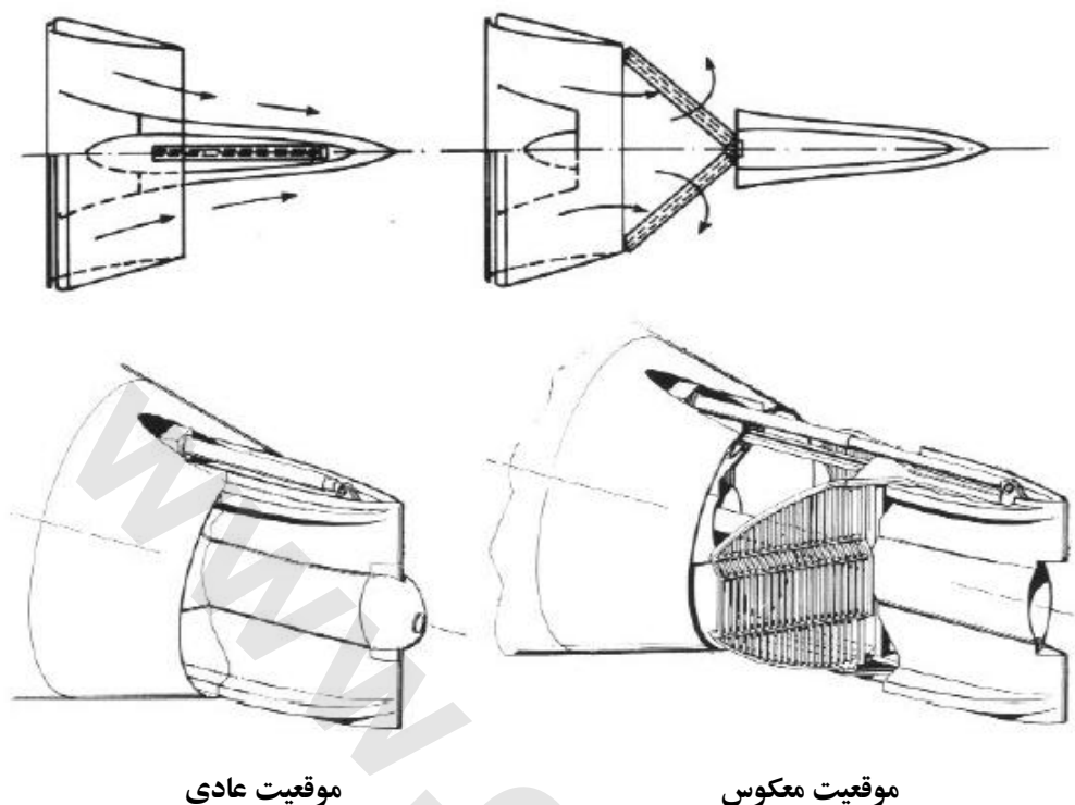
شکل ۱۸-۷ نیروی محوری معکوس برای جریان هسته موتور ، موتور نسبت کنار گذری بالا (General Electric CF6)
