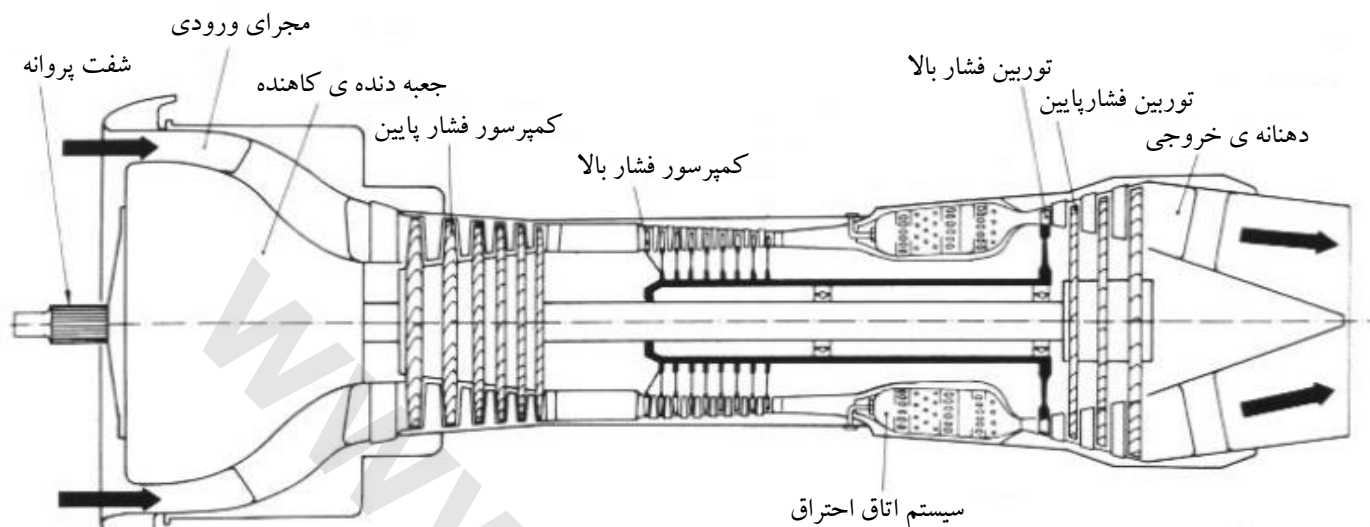
شکل ۱-۵ شماتیک موتور توربوپراپ
