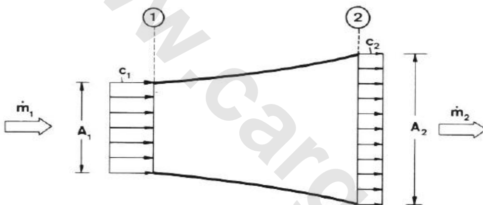
شکل ۲-۶ شرح بقای جرم
