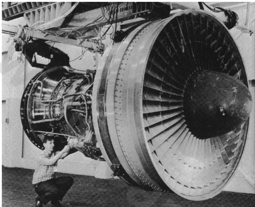
شکل ۲۶ فن قطر بالا ، ویژگی خاصه ی موتور های توربوفن نسبت کنار گذاری بالا می باشد (موتور JT 9D ساخت Pratt & Whitney)
