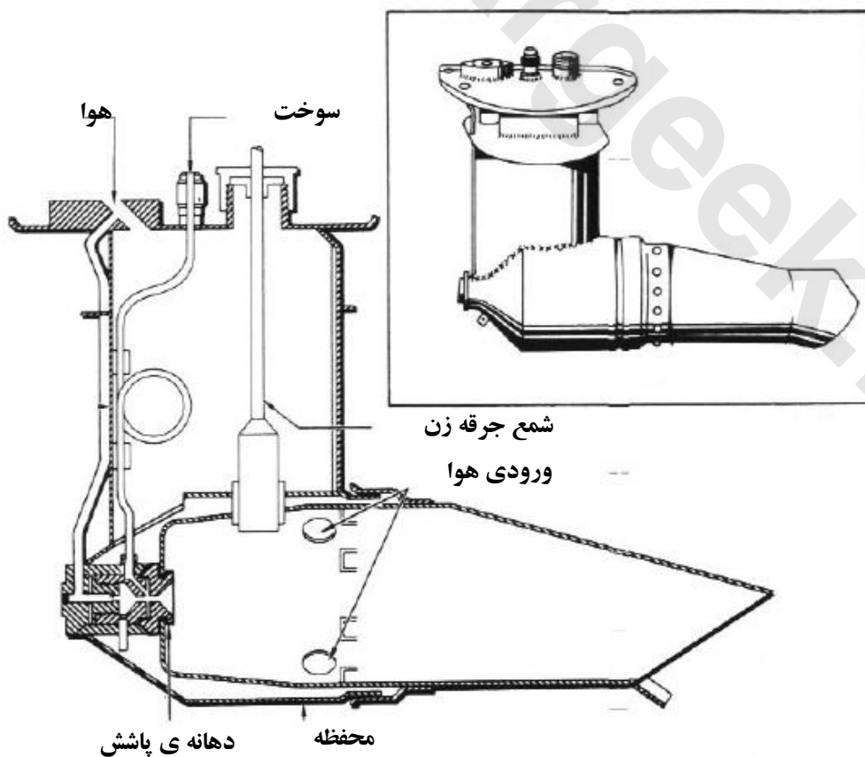
شکل ۸-۸ مشعل کننده ی مشعل (General Electric J79)
