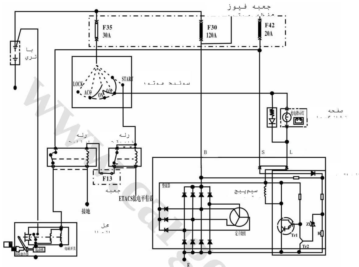
شما تیک دیاگرام برای سیستم استارت و شارژ
