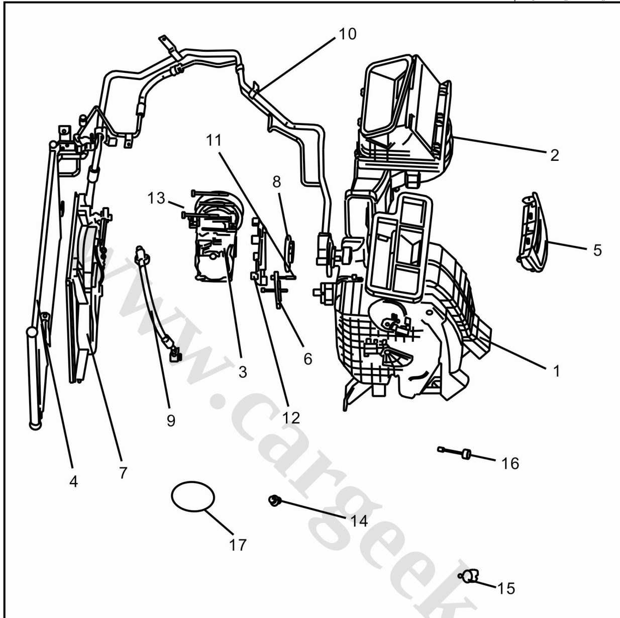
شماتیک دیاگرام قطعات سیستم تهویه مطبوع 1- مجموعه بخاری اوپراتور
