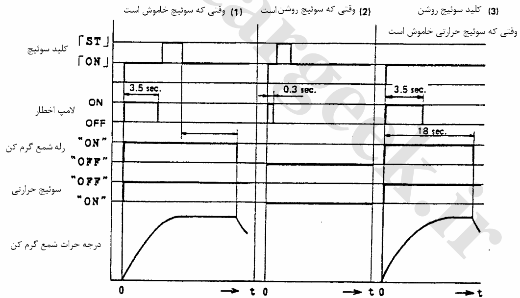
منحنی تایمینگ
