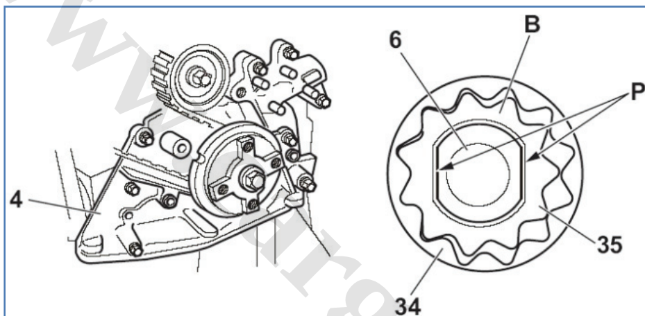
۴- پمپ روغن
