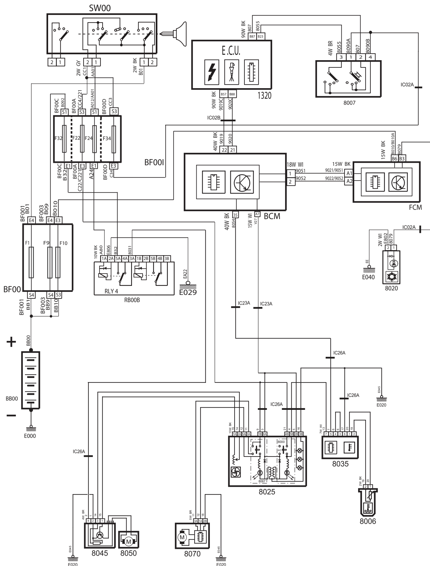
دیاگرام شماتیک مدار سیستم تهویه مطبوع خودروی سمند با سیستم اکوماکس (ECO MUX)
