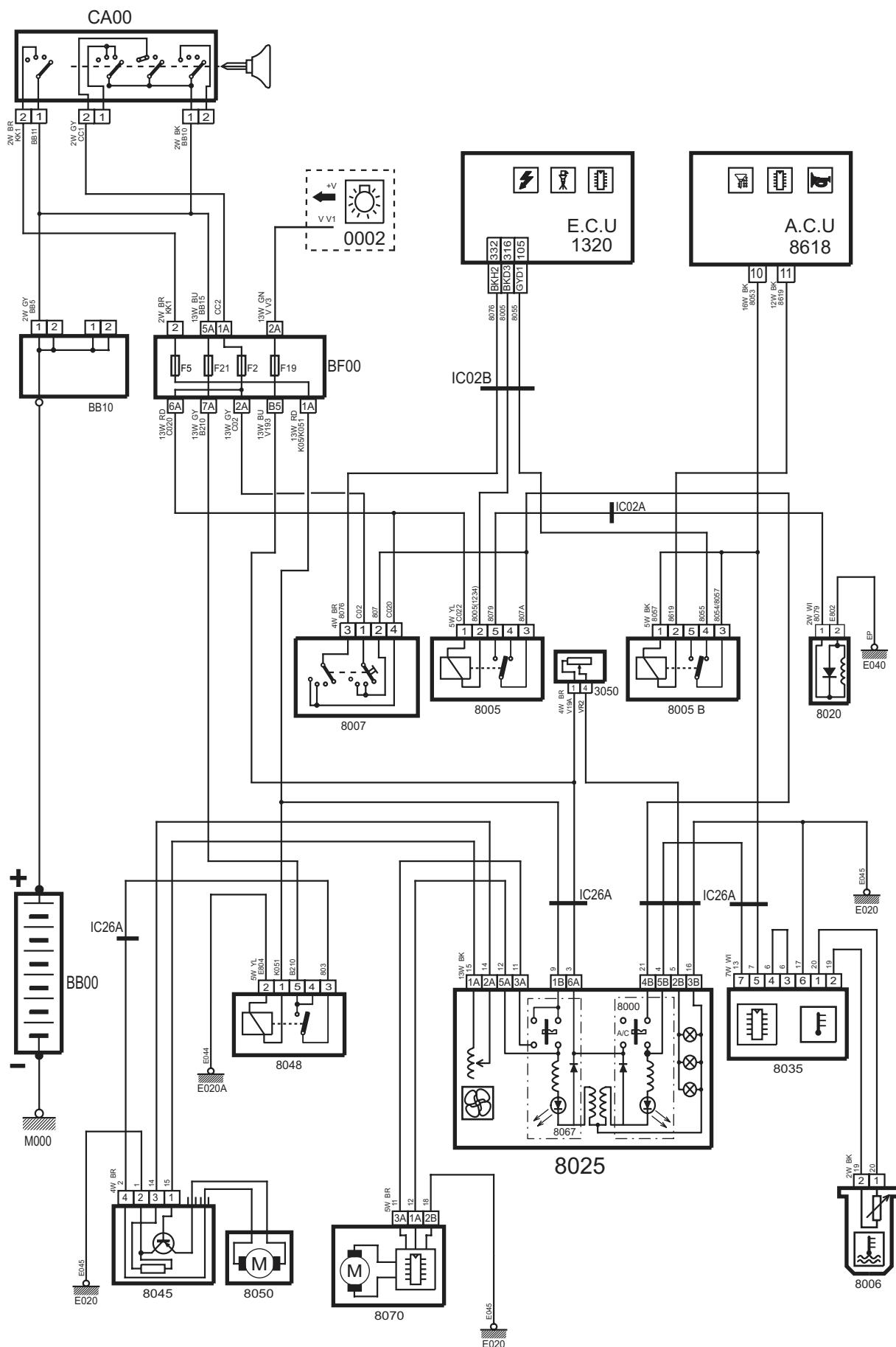
دیاگرام شماتیک مدار سیستم تهویه مطبوع خودروی سمند (وئو، VALEO)
