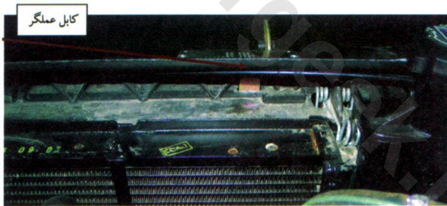
شکل ۱۳- محل نصب عملگر الکتریکی و مسیر عبور کابل عملگر
