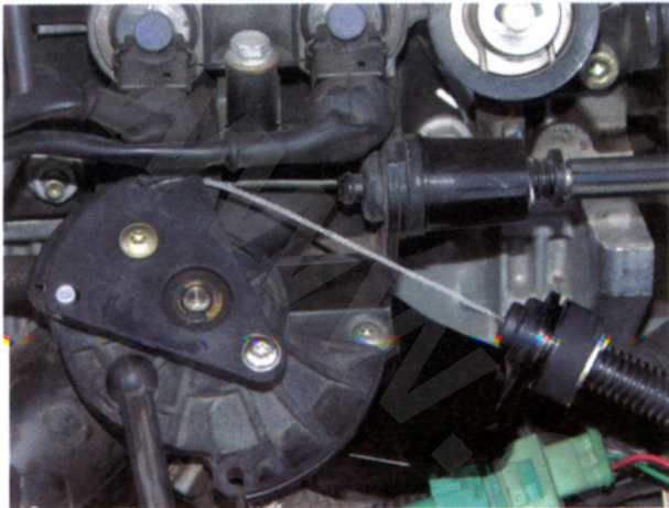
شکل ۱۵- محل نصب براکت کابل عملگر و کوپلینگ تراتل
