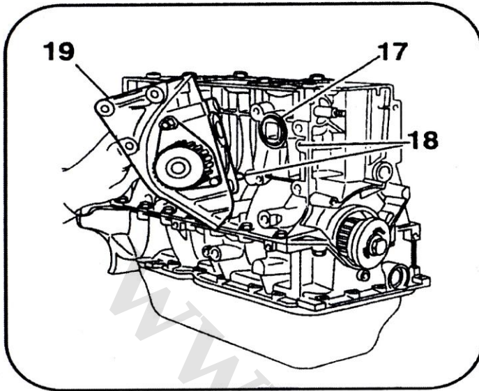
گشتاور پیچ IV110 به میزان 0.5da.Nm گشتاور پیچ M8 به میزان 3 da.Nm
