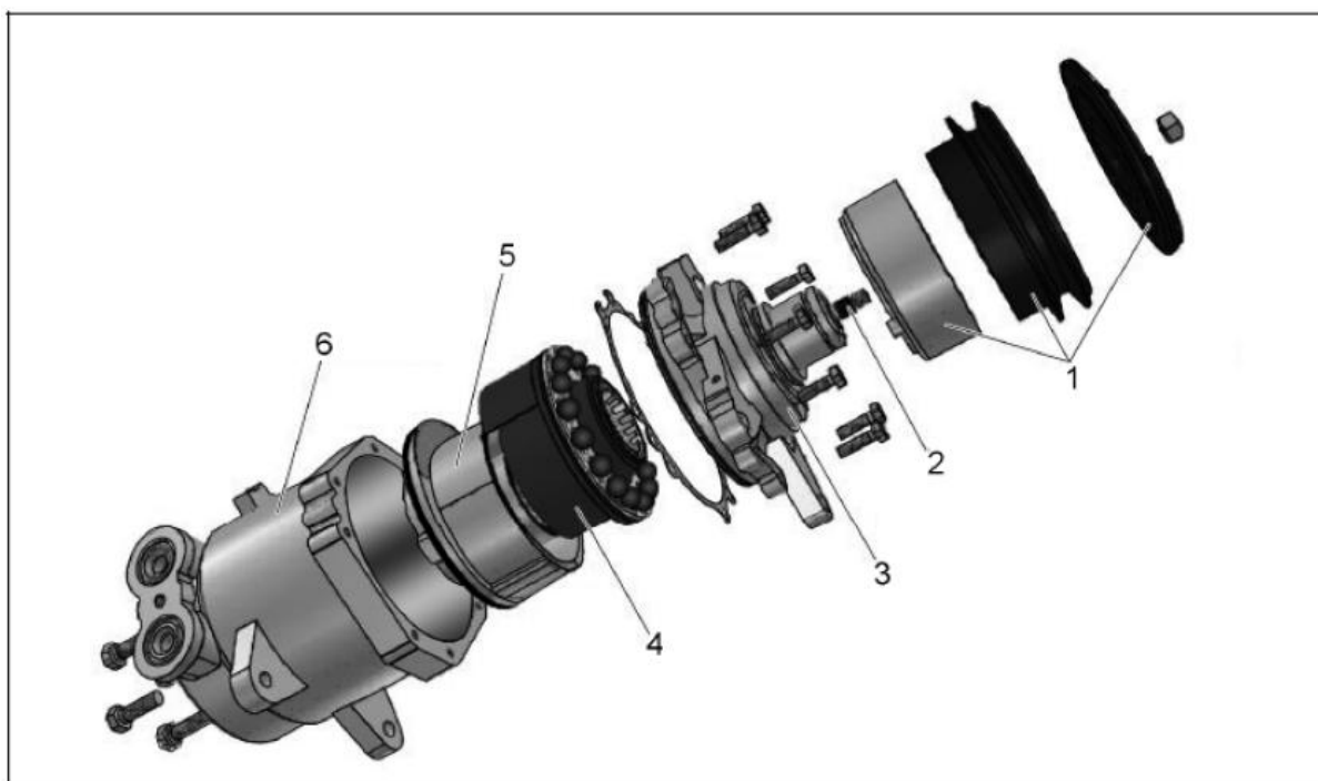
۱- کلاچ ۲- میل لنگ ۳- کاور جلویی ۴- دیسک متحرک ۵- دیسک ثابت ۶- بدنه
