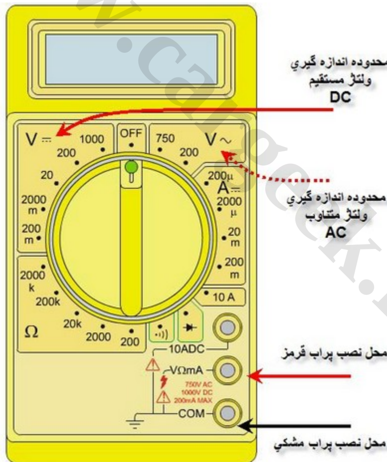
شکل ۹- محل نصب پراب ها و قرار گرفتن سلکتور در مولتی متر دیجیتال
