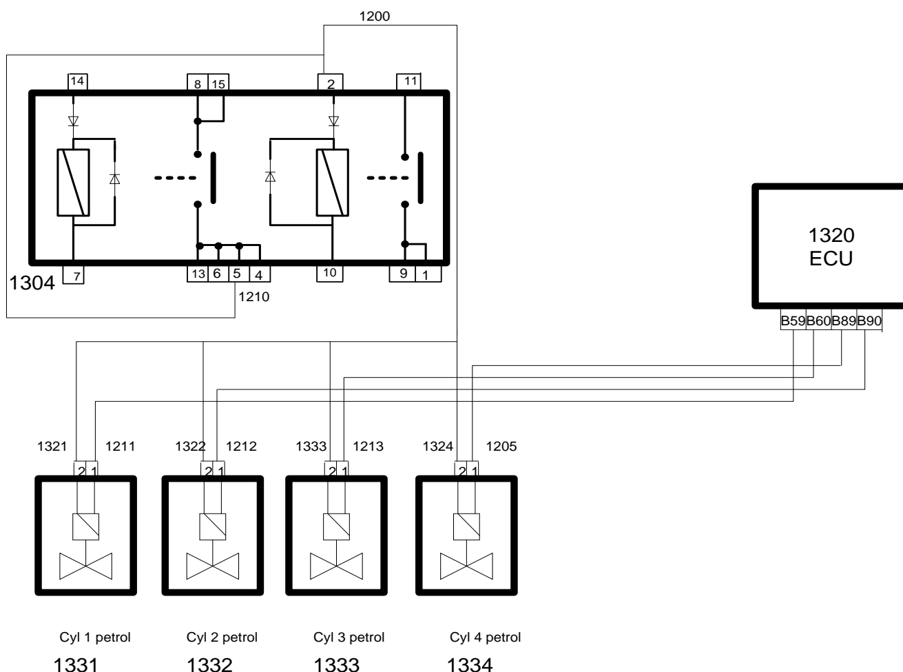
نمودار الکتریکی
