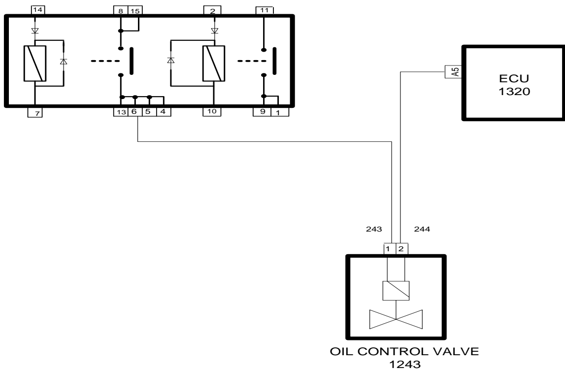
نمودار الکتریکی
