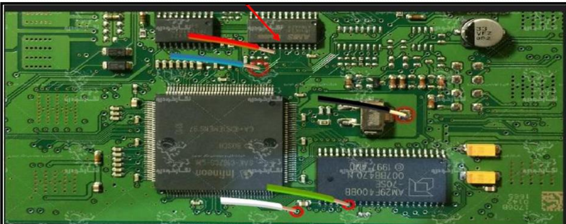
نمای کلی اتصال سیم های فلت رنگی به ایسیو زیمنس بنزینی
