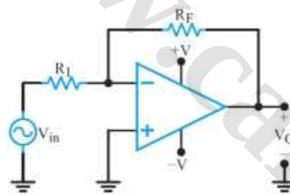
مدار یک تقویت کننده معکوس کننده
