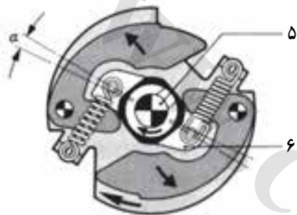
۵- شافت ميل بادامک ۶- بازوهای ميل دلكو \alpha - مقدار زاویه‌ی چرخش
