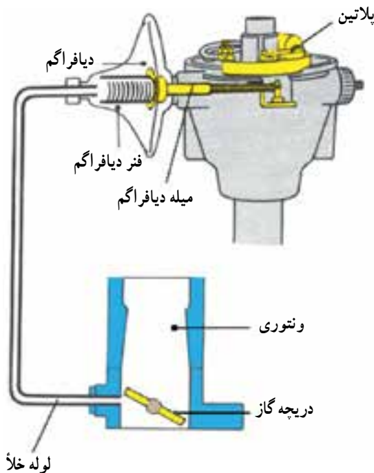
شکل ۱۰-۲۷ مکانیزم دستگاه آوانس خلأ
