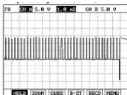
شکل شماره ۵- سرعت سوم دنده D
