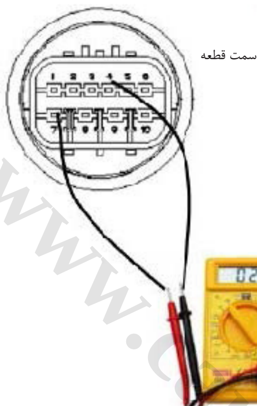
اندازه گیری مقاومت
