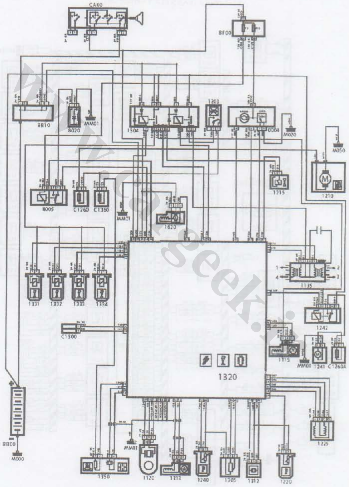
نقشه های شماتیک ECU BOSCH MP7.3 خودروهای پژو پارس ELX و سمند سریر
