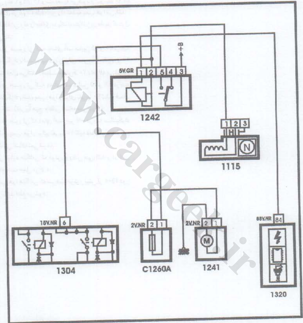
مدار الکتریکی زله پمپ هوا و ECU
