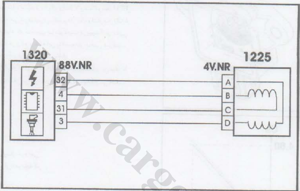
مدار الکتریکی استپر موتور
