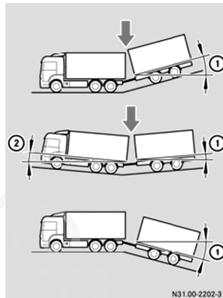
خودروی کشنده با تریلر محور مرکزی (مثال)
