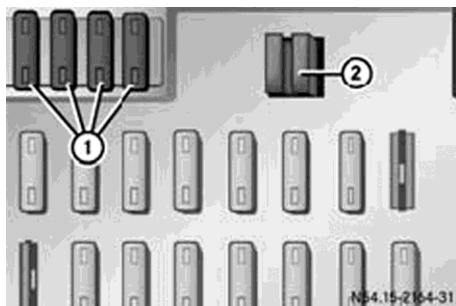
جعبه فیوز اصلی
