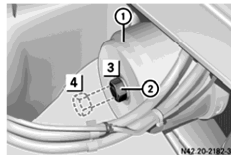
سیلندر فنی ترمز پارک با پیچ آزاد کننده
