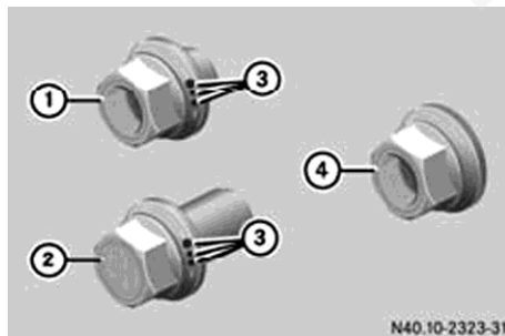
مهره‌های چرخ
