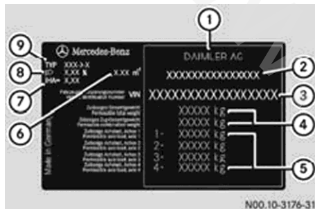
صفحه مشخصات شناسایی خودرو (مثال)
