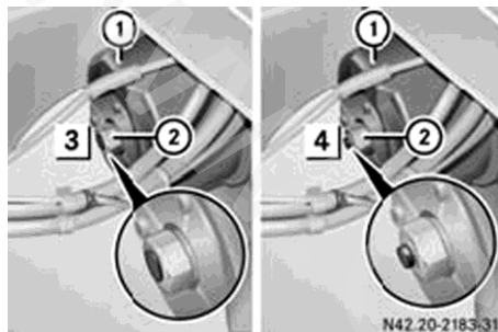
سیلندر فنی ترمز پارک با پیچ آزاد کننده و ضامن آزاد کننده
