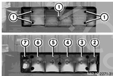
چراغ عقب شش محفظه‌ای - سمت راست
