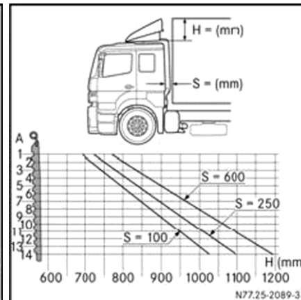
کابین نوع S یا L با بادگیر دو تکه (مثال: کابین نوع L)
