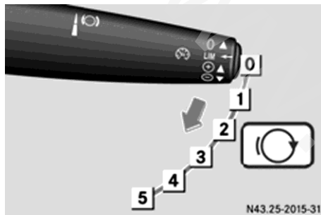
اهرم چندکاره (مثال)
