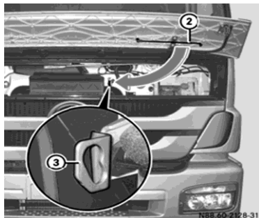
درب سرویس و نگهداری جلوی خودرو بدون پایه نگهدارنده گازی
