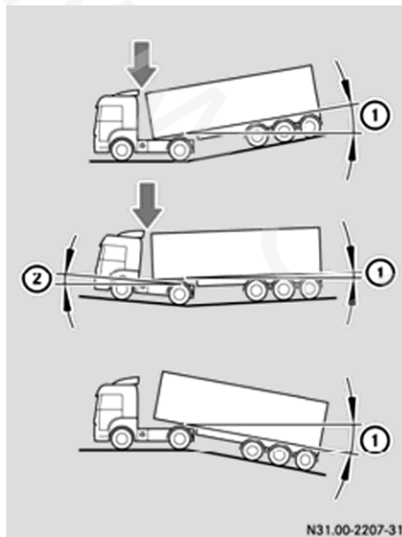
خودروی کشنده با نیمه تریلر (مثال)
