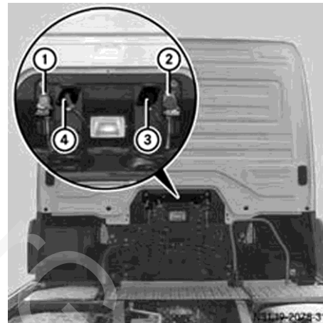
اتصالات نیمه تریلر (مثال)
