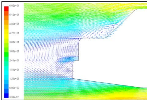
شکل (۹) تزریق هوا از بالای سپر عقب با نرخ 0.5 \text{ Kg/s}
