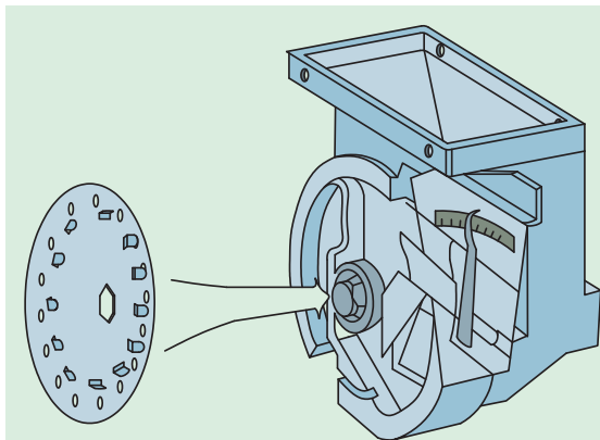
شکل ۳-۴۷. جهت بستن صفحه موزع نیوماتیک
