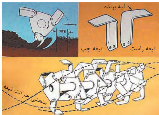
شکل ۱۵-۱. آرایش مارپیچ تیغه‌های گاواهن دوار
