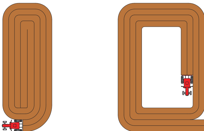
ب- شخم از مرکز به محیط
