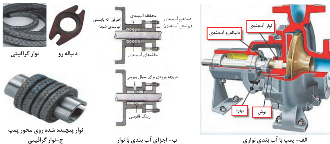
شکل ۵-۵۰. آب بندی پمپ با نوار گرافیتی
