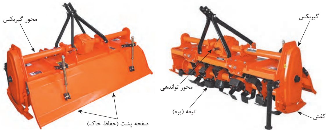
شکل ۱۴-۱. گاواهن دوار (رتیواتور)
