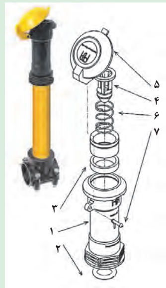
شکل ۳۹-۵. ضامن رایزر و شیر خودکار
