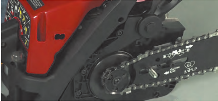
شکل ۴-۵۵. کلاچ گریز از مرکز
