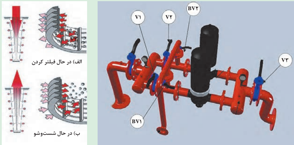
شکل ۶۱-۵. شیرهای روی صافی دوقلو دیسکی
