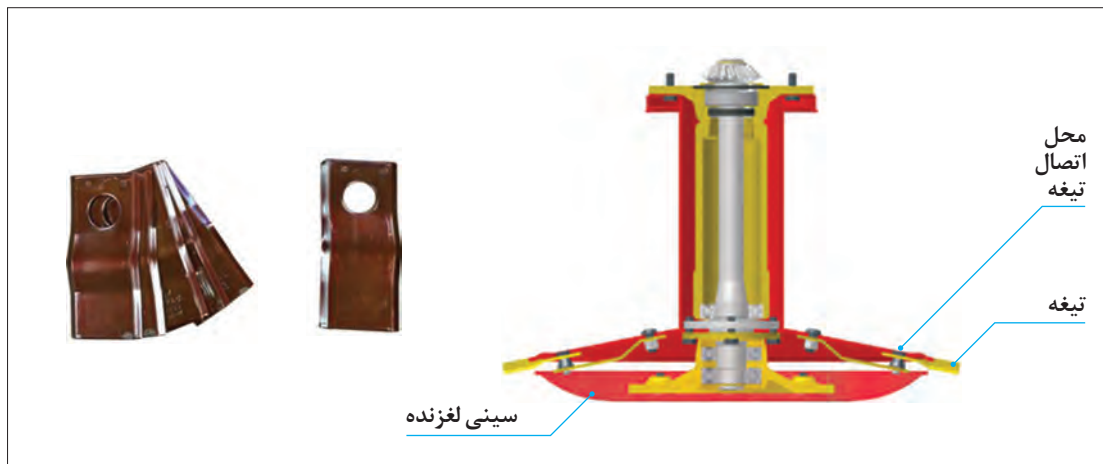
شکل ۴- تیغه و محل قرارگیری آن روی استوانه
