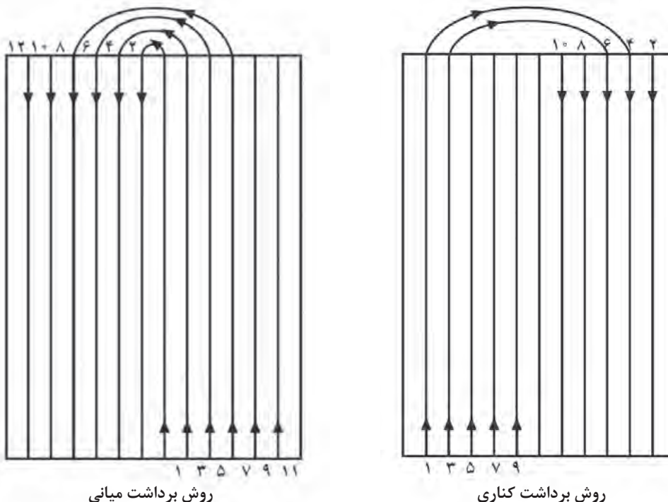
شکل ۵۷ - مسیر حرکت چپر هنگام برداشت
